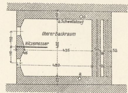
D. Horizontalschnitt VII.VII.
