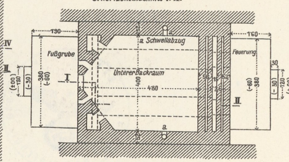
C. Horizontalschnitt V.VI.
