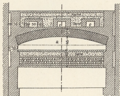
C. Querschnitt V.VI.
