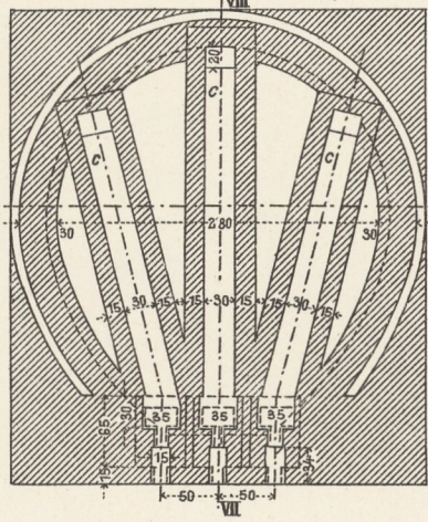
B. Horizontalschnitt III.IV durch die Dippelzüge.
