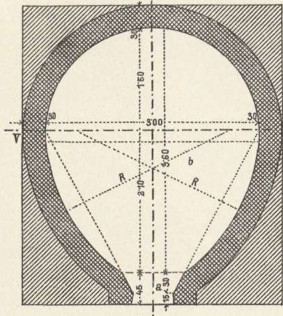
A. Horizontalschnitt I.II über der Herdsohle.
