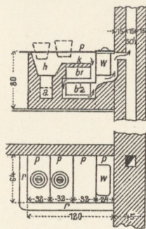
5. Kleiner gemauerter Tischherd.
