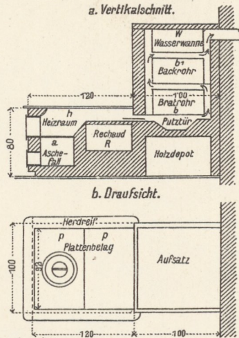
3. Sparherd, kleiner gemauerter Tischherd.
