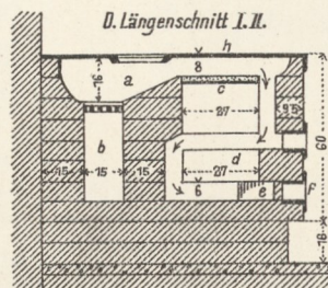
5. Kleiner gemauerter Tischherd.
