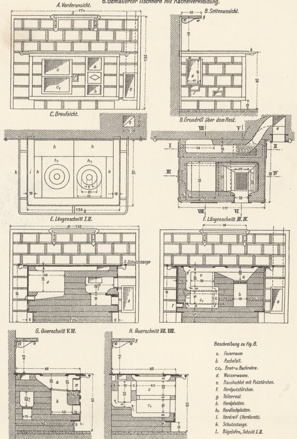
6. Gemauerter Tischherd mit Kachelverkleidung.
