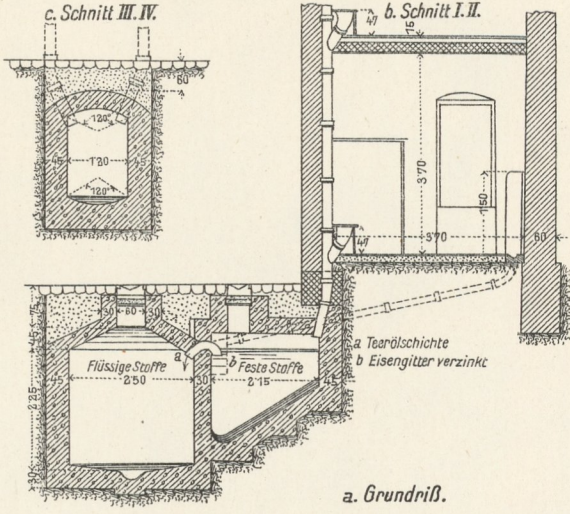
2. Abortanlage mit 4-Sitzen und runder Senkgrube zur Scheidung der festen u. flüssigen Stoffe.
