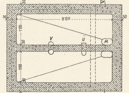
f. Detailschnitt VII. VIII.
