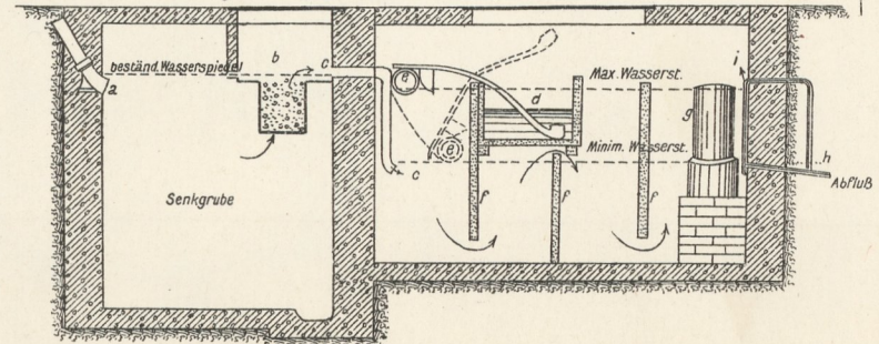
mit automatischer Entleerung und Desinfizierung. System Krölein.
