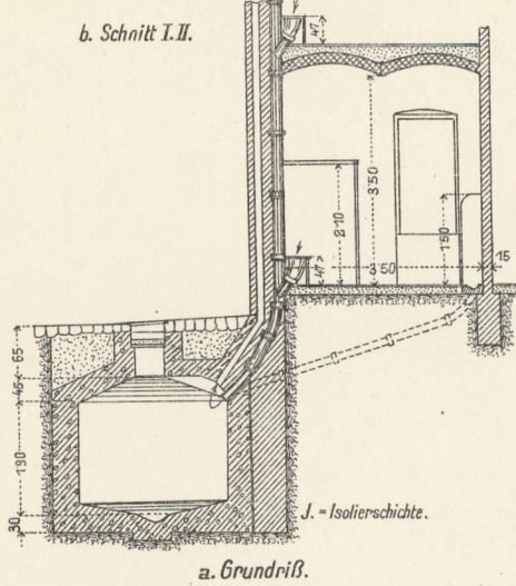
1. Abortanlage mit 4-Sitzen und runder Senkgrube.
