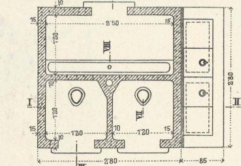
b. Grundriß.
