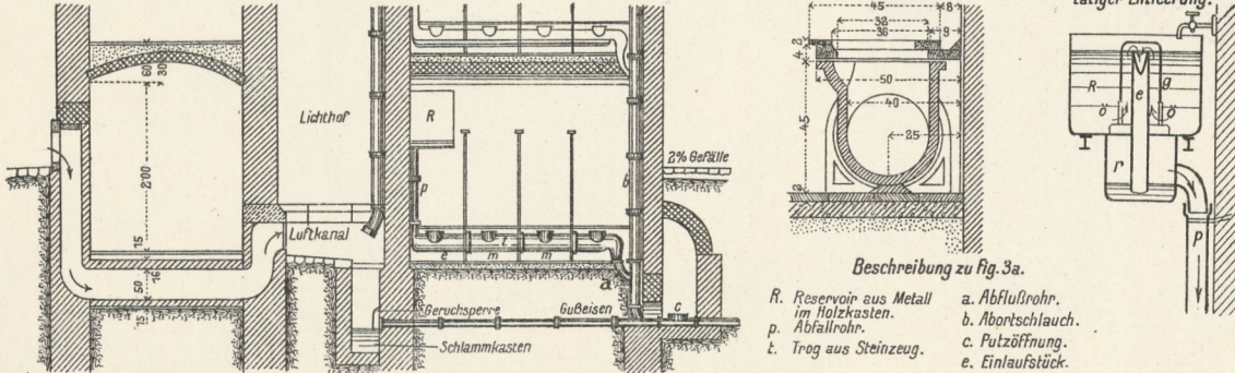
d. Längenschnitt V. VI. durch den Trog.
