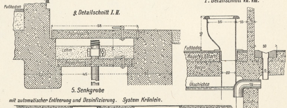
f. Detailschnitt VII. VIII.
