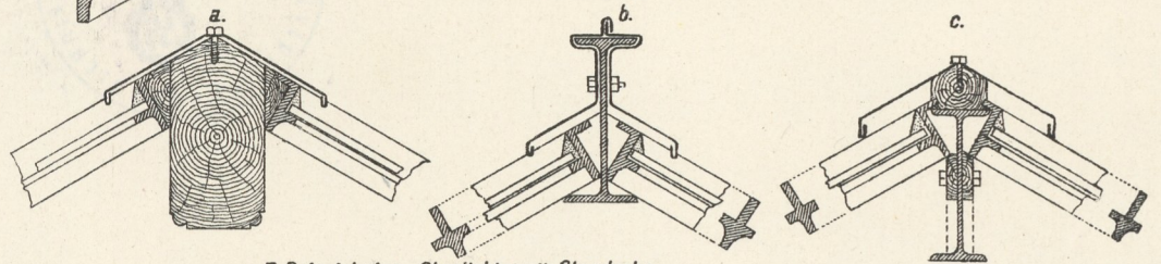
7. Beispiel einer Oberlichte mit Glasdecke.
