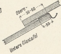
9. Schweißrinne bei den Übergreifungsstellen.
