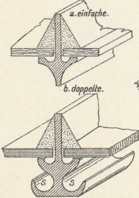
8. Fenstereisen mit Schweißrinnen.
