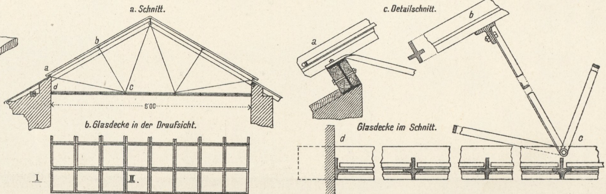
7. Beispiel einer Oberlichte mit Glasdecke.
