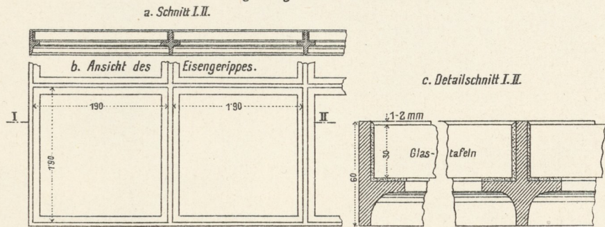
4. Verglasung von Fußbodenoberlichtern.
