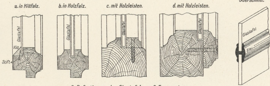
3. Befestigung der Glastafeln auf Fasseneisen.
