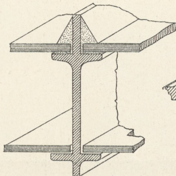
10. Verglasung auf Fenstereisen mit doppeltem Falz.
