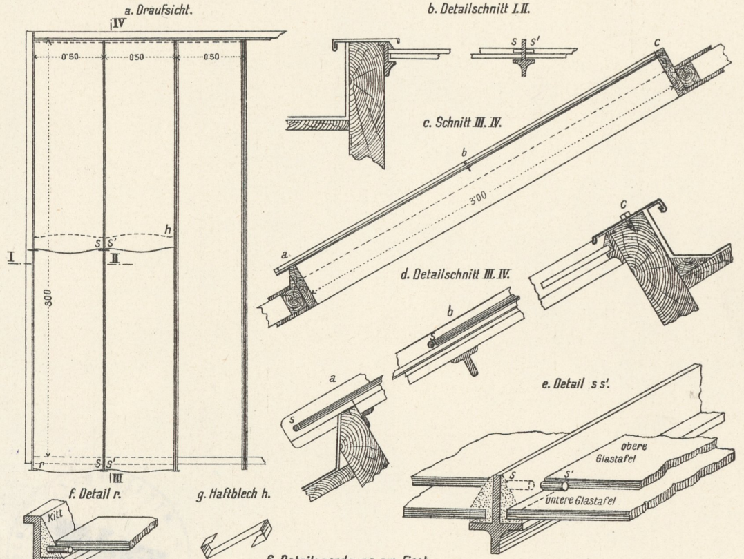
6. Detailanordnung am First.
