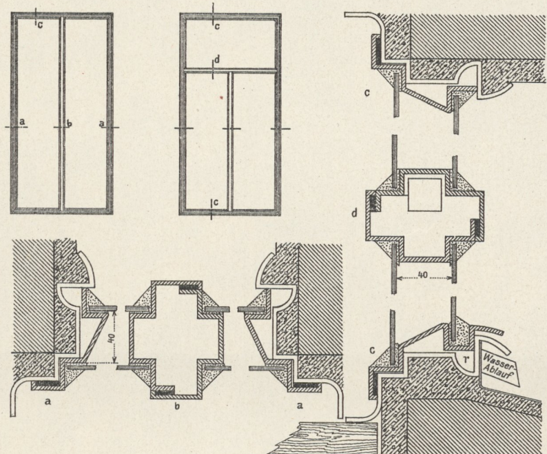
Fig. 3. Zweiflügelige Fenster mit und ohne Oberlichte, Gillar-Fenster.
