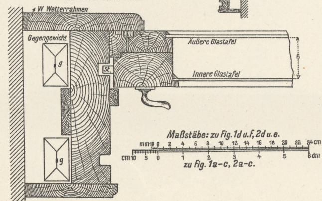
2d. Detailschnitt I. II.
