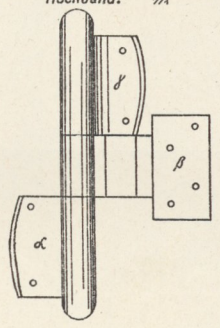
1e. Dreilappiges Fischband.
