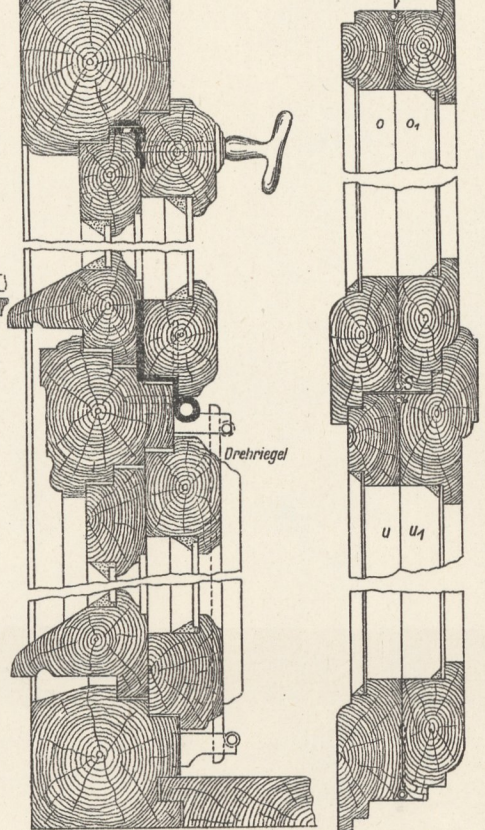
1f. Detailschnitt III. IV.
