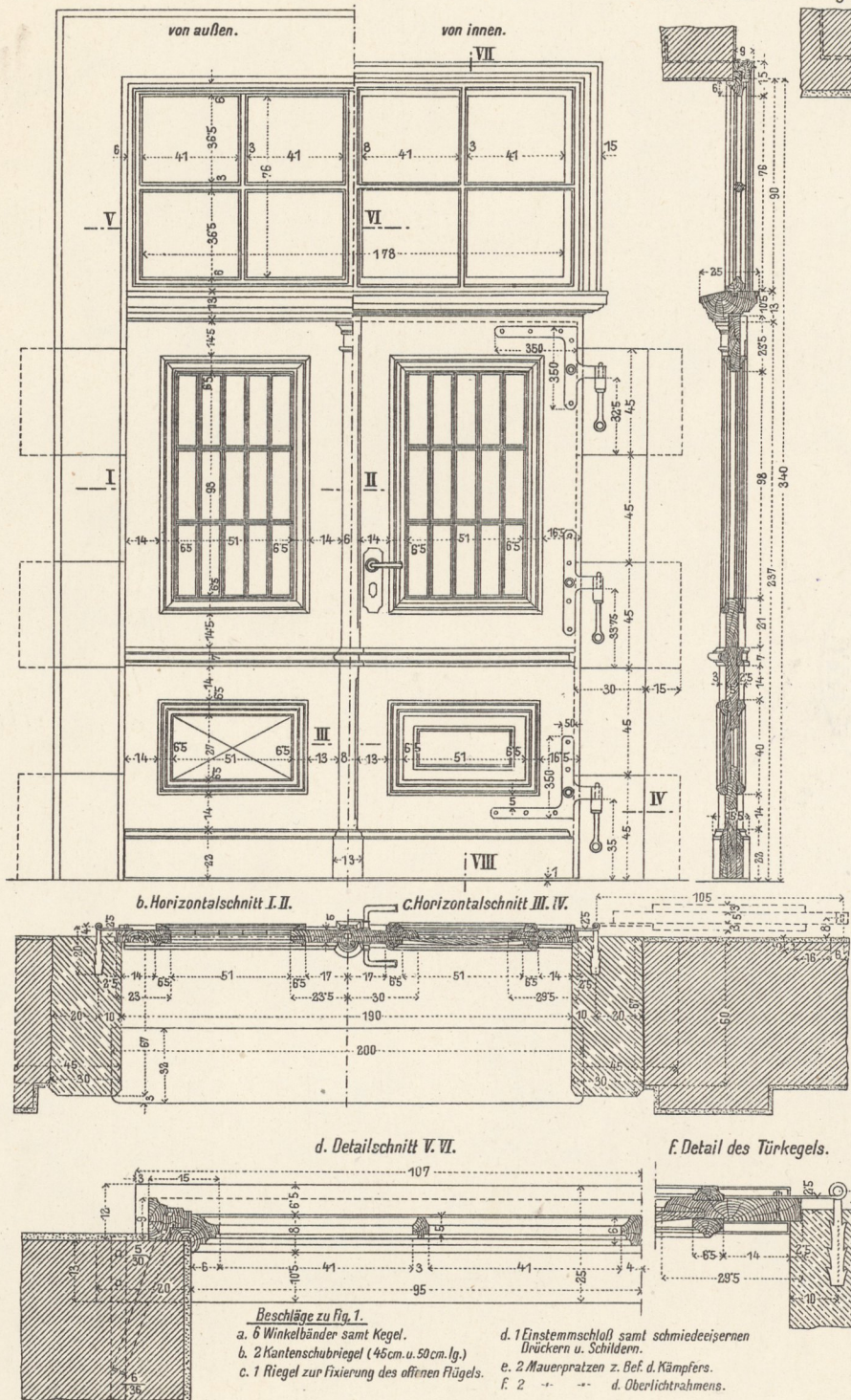
1. Türen mit steinernem Gewände. a. Ansicht.
