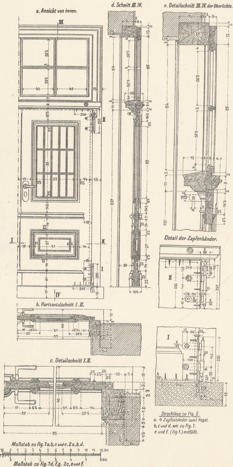
2. Alternative für Türen mit Holzstock und Zapfenbeschlägen.
