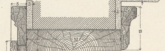
2f. Details zum Türsturz.
