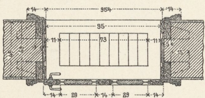
1d. Details zum Hörenschnitt.
