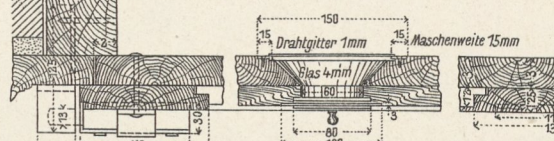
2f. Details zum Türsturz.
