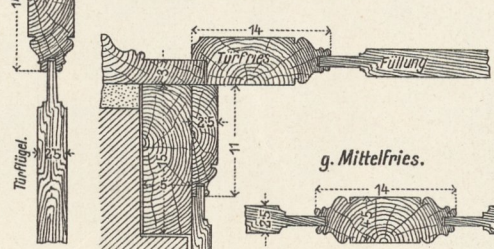
1f. Details zum Grundriß.
