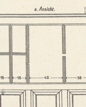
24. Abteilungswand mit Verglasung.
