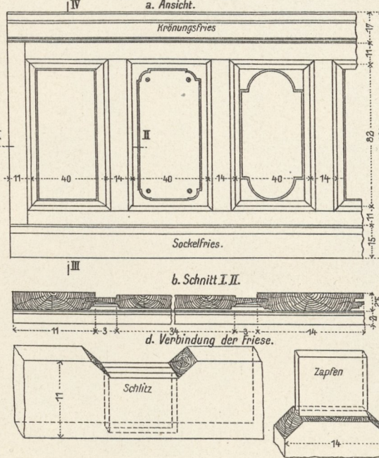
22. Wandvertäfelung.
