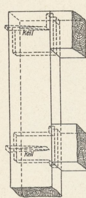
15. Nutzapfen mit Keil.
