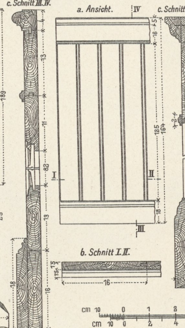
23. Wandvertäfelung.
