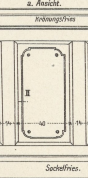
22. Wandvertäfelung.
