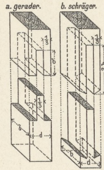
15. Nutzapfen mit Keil.
