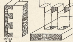
8. Vergabelung.
