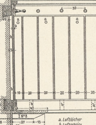
25. Wandverkleidung in Bäderräumen.
