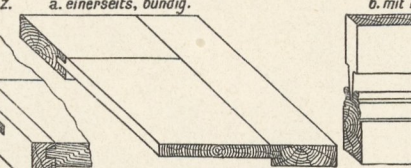
5. Verbindung mit Rahmen, Fries und Füllungen.
