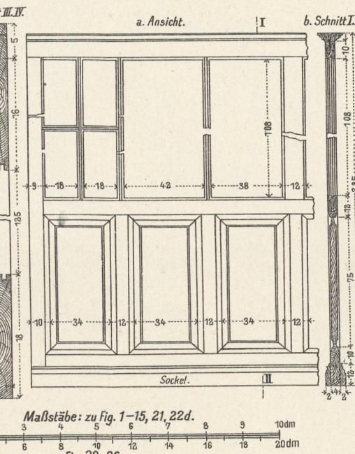
24. Abteilungswand mit Verglasung.
