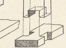
9. Schlitzzapfen.
