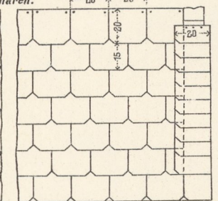
9. Universal-Doppeldachziegeldach von Lannach.
