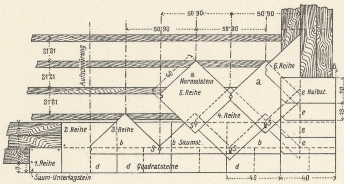
1a. Normalstein. 1b. Saumstein. 1c. Saumunterlagstein. 1d. Quadratstein.
