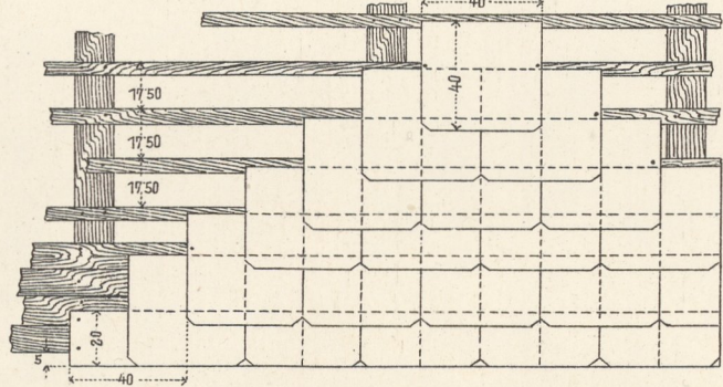
b. auf einer Einlattung.
