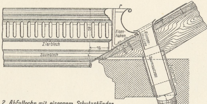
2. Abfallrohr mit eisernem Schutzständer.
