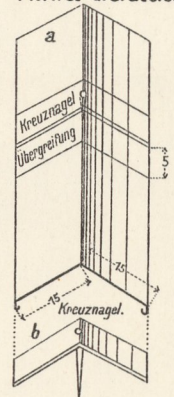
14. First- u. Gratblech.
