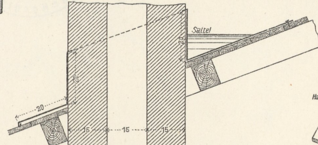
13. Brand- und Feuermauereindeckung.
