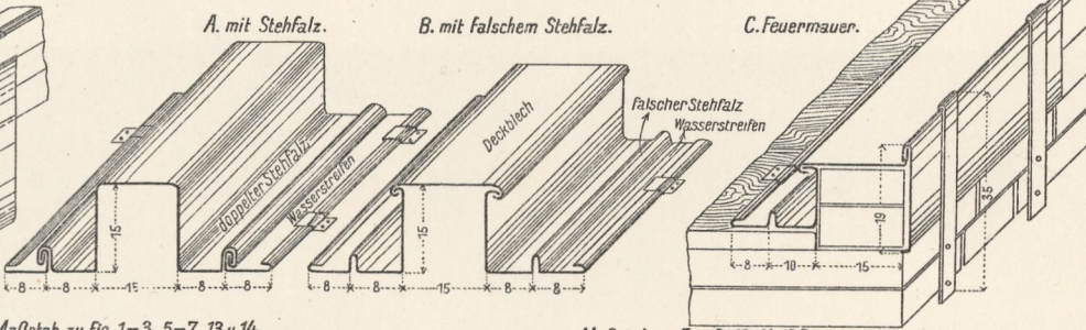
13. Brand- und Feuermauereindeckung.
