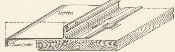
10. Giebelsaum mit falschem Stehfalz.
