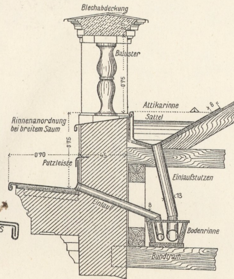
7. Attikarinne.
