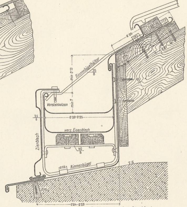
8. Kehlrinne bei Sheddächern.
