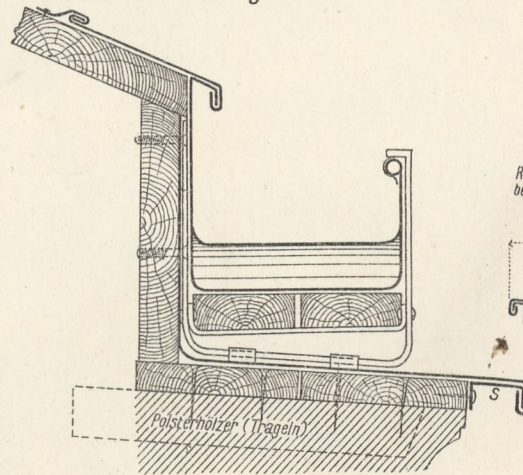
6. Kastenrinne als aufliegende Stehrinne.
