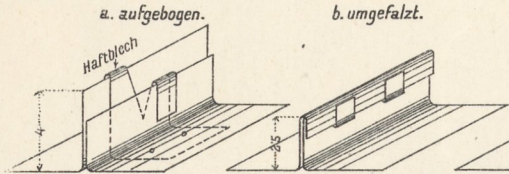
3. Doppelt stehender Falz.
