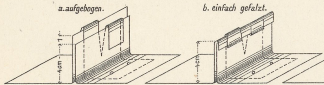
3. Doppelt stehender Falz.
