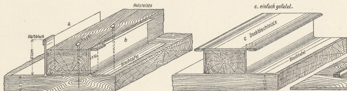
6. Französische Eindeckungsmethode.
