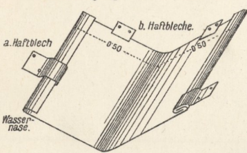
7. Befestigung bei Zinkblechrinnen.
