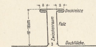
8. Schiefefalz.
