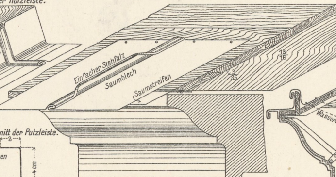
13. Dachsaum.
