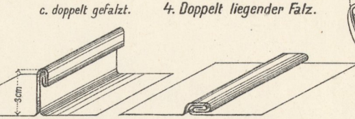
5. Deutsche Eindeckungsmethode.
