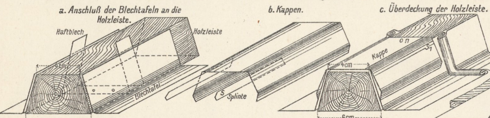
7. Befestigung bei Zinkblechrinnen.
