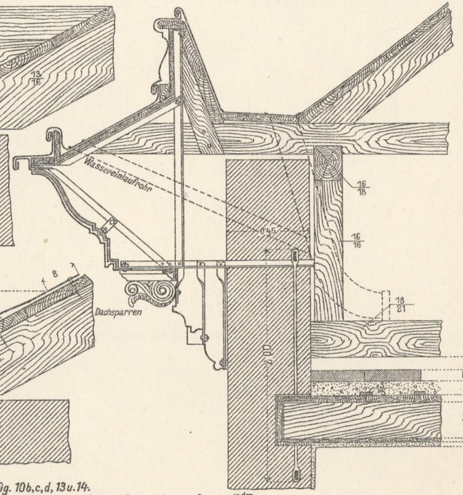
15. Hauptgesimse mit Zinkornament und Eisenkonstruktion.
