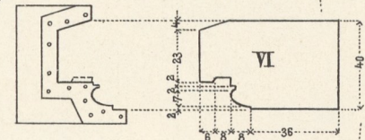
7. Kontraschablone.
