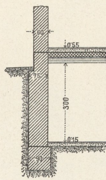
3. Isolierung der Kellerumfassungsmauern.
