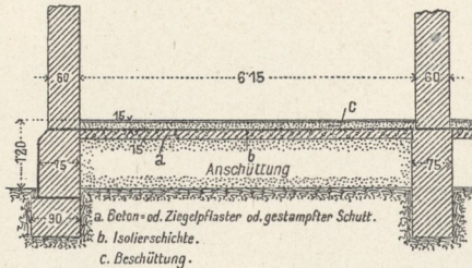
2. Horizontale Isolierung mit Asphaltfilzplatten über die ganze verbaute Fläche.
