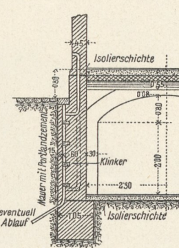
4. Isolierung der Kellermauern mit vorgelegtem Luftschlitz.
