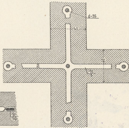
11. Kreuzanker.
