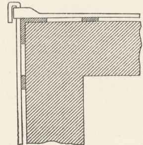
21. Eckanker.
