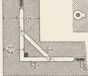
10. Eckanker.
