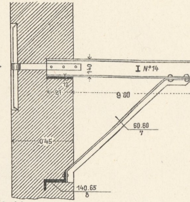
6. Balkonträgerverankerung.
