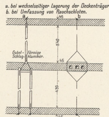
19. Anordnung der Zuganker.
