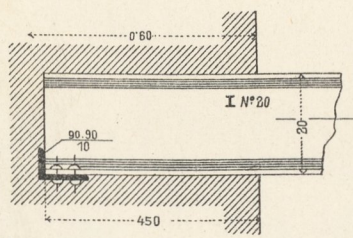
5. Auflager, gleichz. Zuganker.
