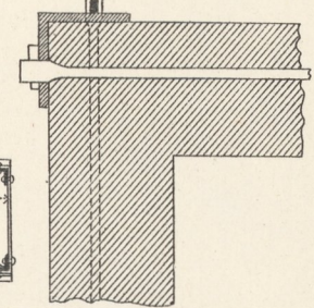
23. Eckanker.
