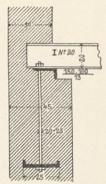
7. Träger-Auflager, gleichz. Druckanker.
