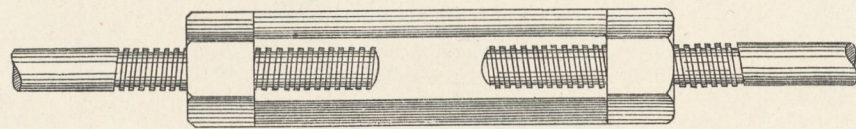
16a. Muffenschloß (Holländische Schraube) mit Spannstangen.
