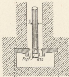
3. Lösbare Verankerung mit Druckplatte.
