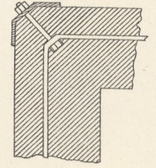
23. Eckanker.
