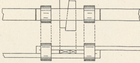
18. Gewöhnliches Keilschloß. (Siehe Fig. 9 Taf. 38.)
