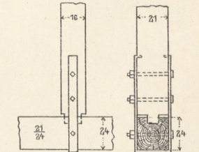
9b. Detail II zu Fig. 9.
