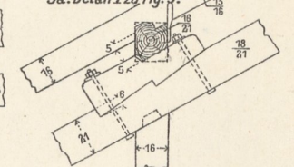
9b. Detail II zu Fig. 9.
