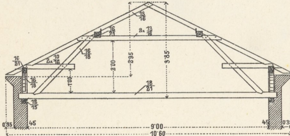
7. Flugstuhl, normale Ausführung.
