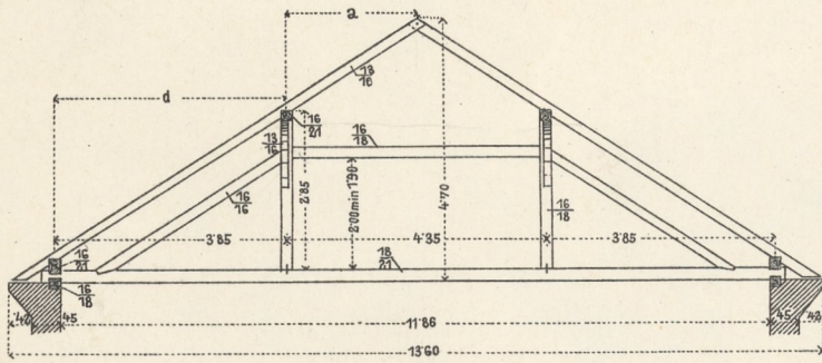
2. Doppelstuhl, Abart a.
