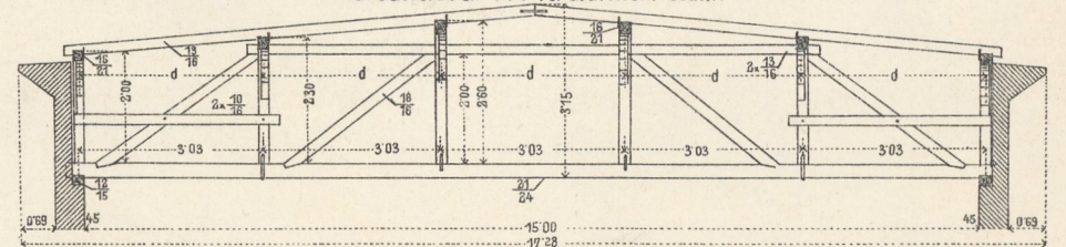
12. Satteldach mit verstärktem Stuhl.
