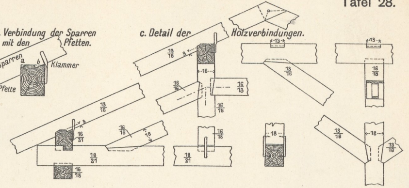
4. Doppelstuhl, Abart c.
