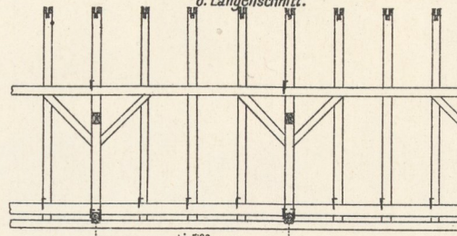
1. Doppelstuhl, normale Ausführung. b. Längenschnitt.
