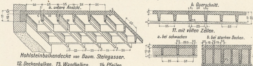
Querschnitt.
