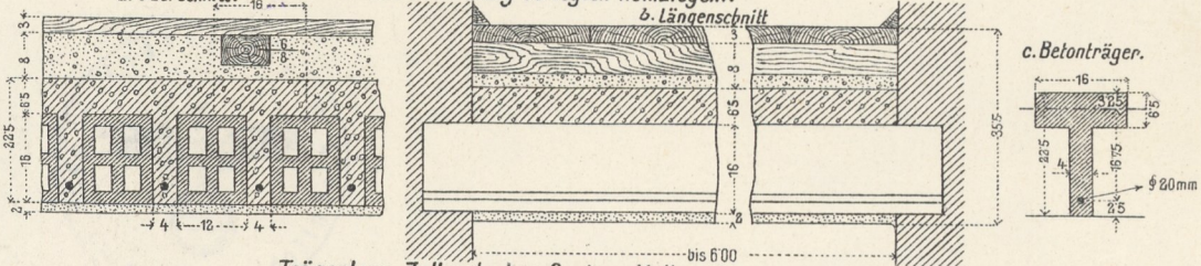
a. Querschnitt.
