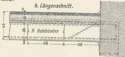
b. Längenschnitt.
