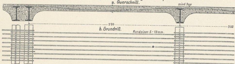
a. Querschnitt
