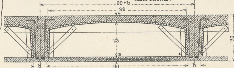
Querschnitt.
