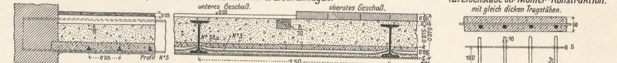
11. Flachdecken, System Monier (Patent G. A. Wayß Komp.)
