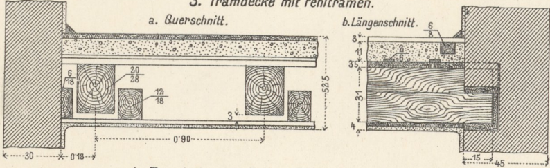
4. Tramdecke mit Fachausfüllung (Einschubdecke)
