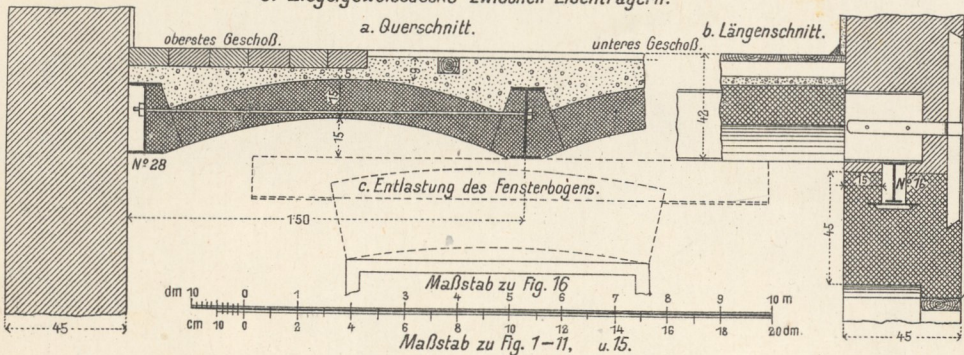
6. Ziegelgewölbsdecke zwischen Eisenträgern.
