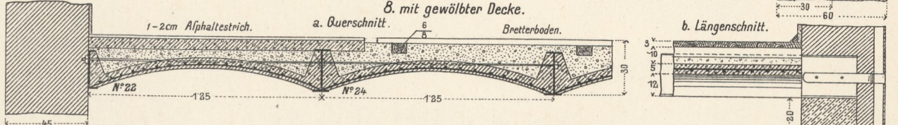
9. mit gewölbter Decke und Betonestrich. a. Querschnitt.
