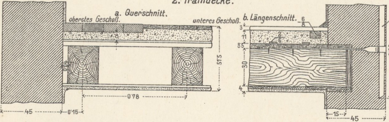
3. Tramdecke mit Fehlträmen.
