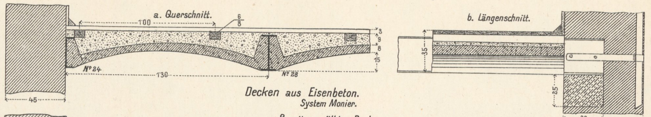
8. mit gewölbter Decke.
