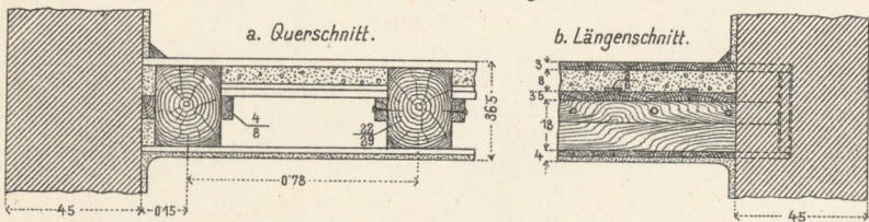
5. Tramdecke zwischen Eisenträgern.
