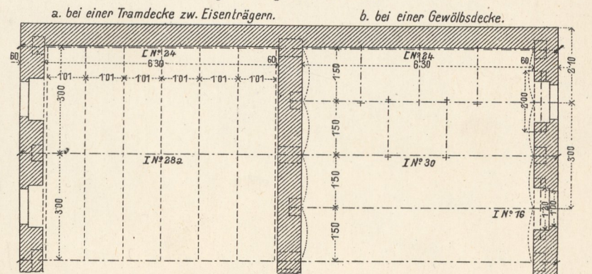
16. Austeilung der Träger im Grundriß.
