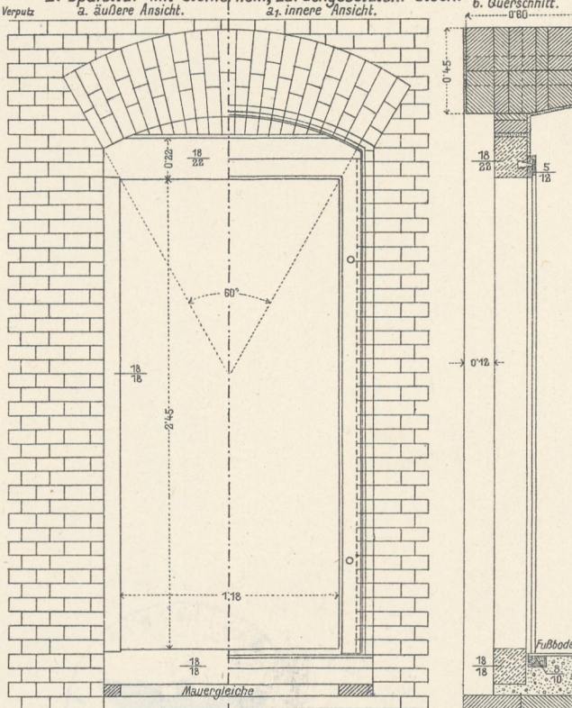
c. Grundriß.
