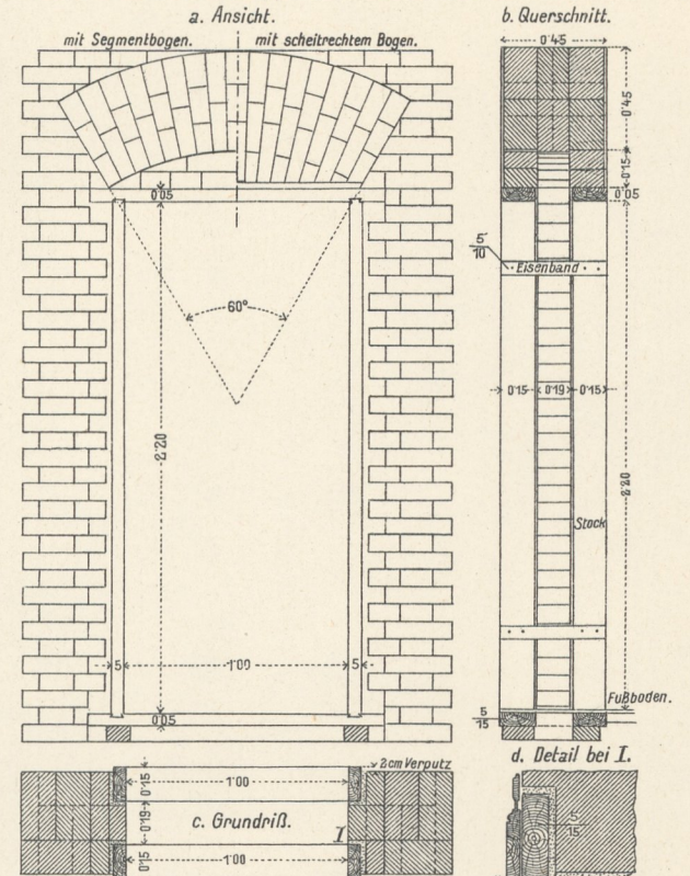
9. Hauseingangstür.
