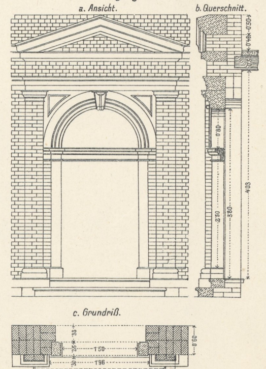
9. Hauseingangstür.
