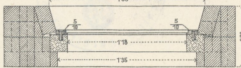
8. Tor mit Quaderverkleidung.
