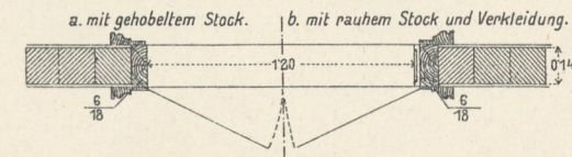
5. Futtertür bei 15 oder 30cm breitem Stock.
