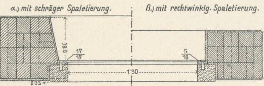
4. Spalettür mit hölzernem Stock.
