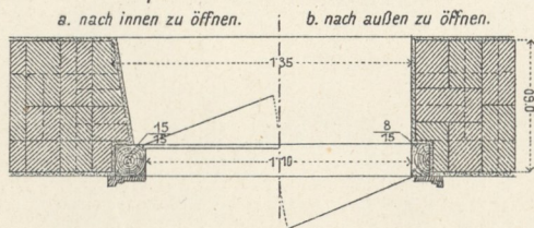
5. Futtertür bei 15 oder 30cm breitem Stock.
