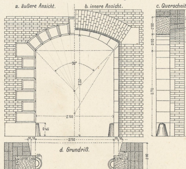
8. Tor mit Quaderverkleidung.
