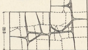
2. Cyklopenmauerwerk.
