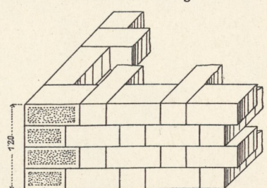
7. Quaderverkleidung.
