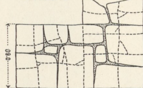
3. Schichtenförm. Bruchsteinmauerwerk.
