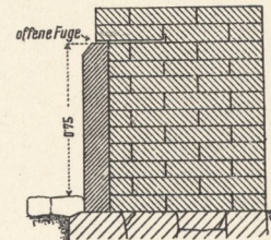
Sockelverkleidungen.
