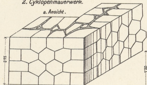
2. Cyklopenmauerwerk.
