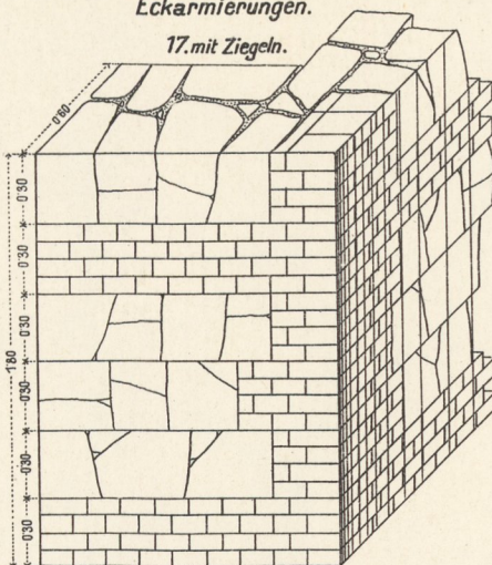
Eckarmierungen.
