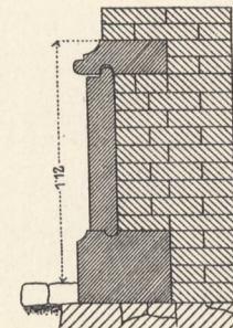
22. mit Quadern.
