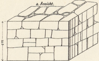
1. Ordinäres Bruchsteinmauerwerk.
