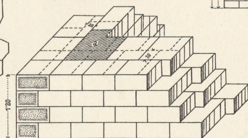
7. Quaderverkleidung.
