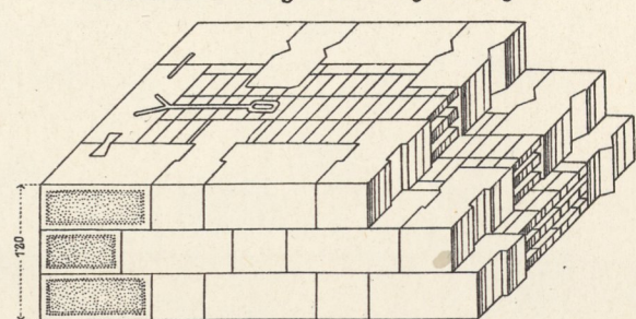
12. Kranztau.
