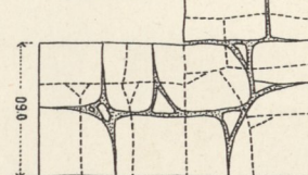
9. Donnerkeil.
