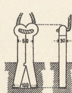
15. Hebelklaue.
