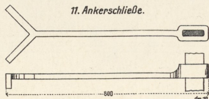
11. Ankerschließe.
