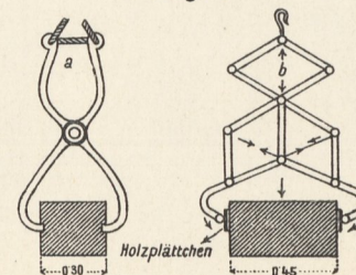
16. Zangen.
