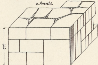
3. Schichtenförm. Bruchsteinmauerwerk.
