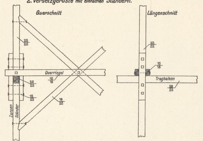
Bewegliche Gerüste.
