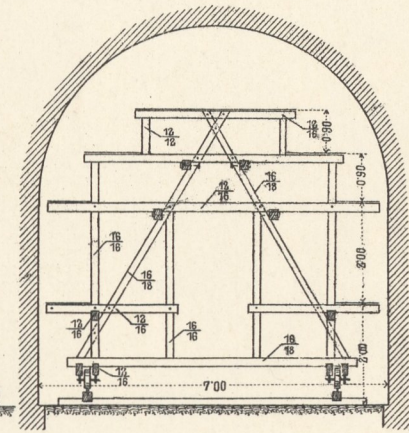
5. Gerüstbrücke.
