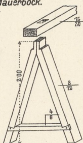
2. Zerlegbarer Mauerbock.
