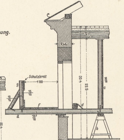
12. Ausschüßgerüste, für Demolierungen etc.
