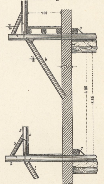
12. Ausschüßgerüste, für Demolierungen etc.
