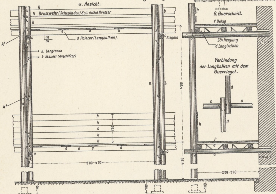
5. Langtennengerüste mit durchlauf. Tragbalken.
