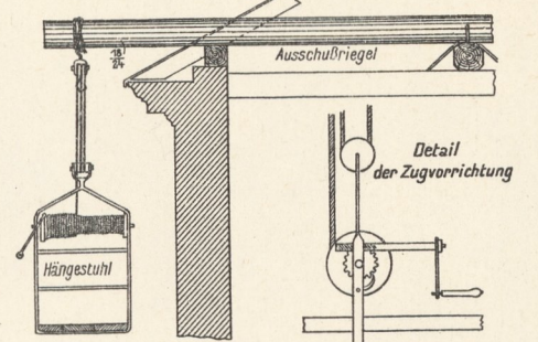
11. Ausschüßgerüste.
