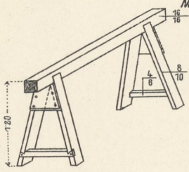
1. Gewöhnlicher
