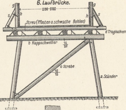
6. Laufbrücke.
