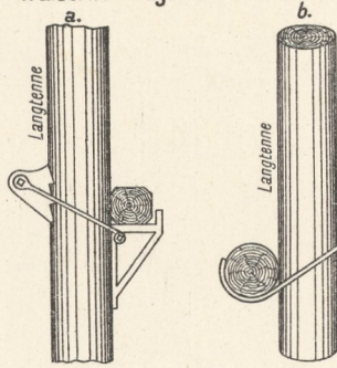
7. Eiserner Träger für Gerüststöcke.
