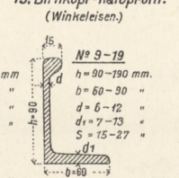
19. Birnkopf-Halbprofil. (Winkelisen).
