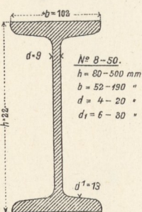
14a. Träger N° 22a.
