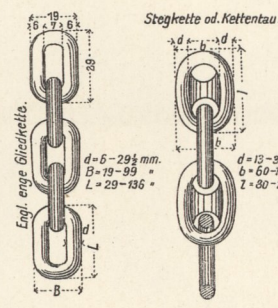
31. Lasketten.
