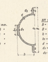
21. Quadrant- oder Viertelkreiseisen.
