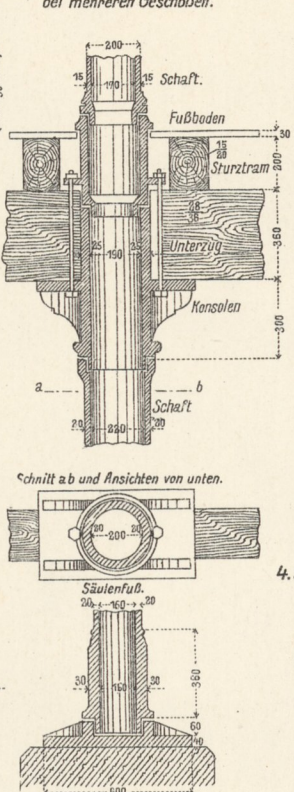
2. mit Konsolen für Holzdecke bei mehreren Geschossen.
