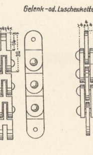
32. Triebketten.
