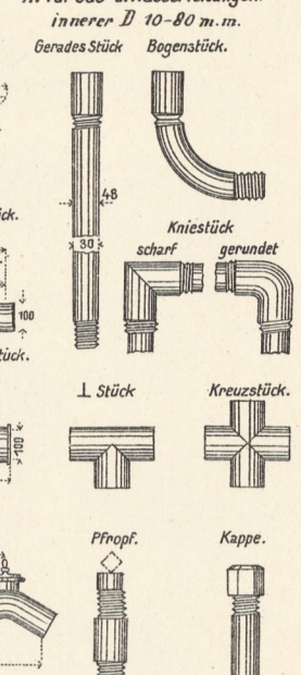
11. Für Gas- u. Wasserleitungen. innerer D 10-80 m. m.
