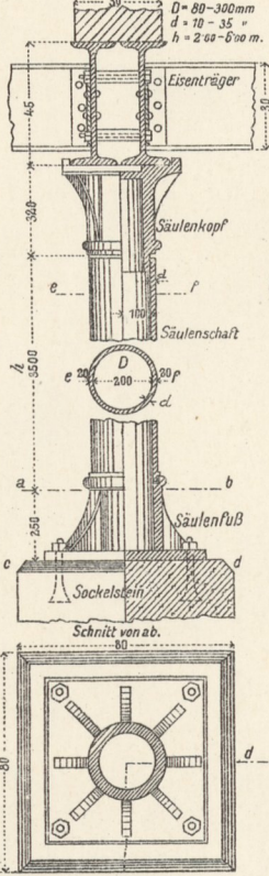
1. Gußeisener Säulen.
