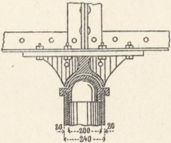
4. Säulenkopf bei Eisenkonstruktion.
