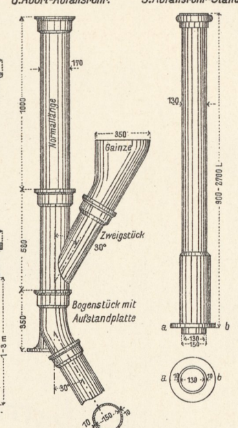
8. Abort-Abfallsrohr. 9. Abfallsrohr-Ständer.
