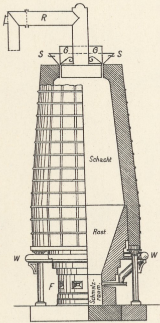
1. Hochofen.
