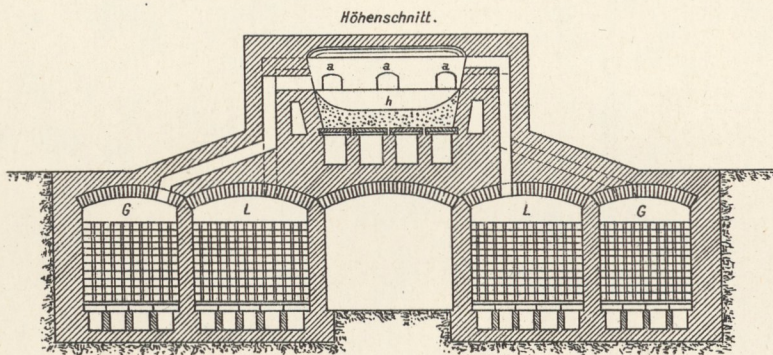
4. Simens-Martinofen.
