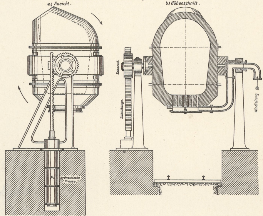
3. Konverter beim Bessemerprozeß.
