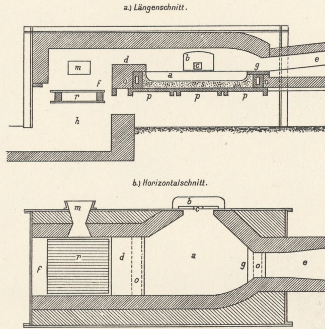
2. Flammofen zum Puddelprozeß.
