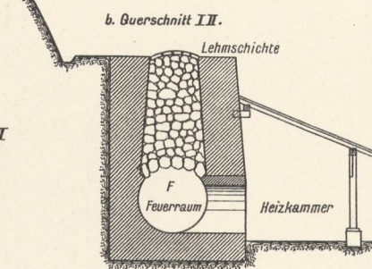
10. Kalkofen mit unterbrochenem Betriebe.
