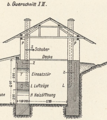
6. Gemauerter Ziegelfofen.
