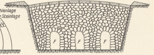
9. Kalk-Grubenofen.
