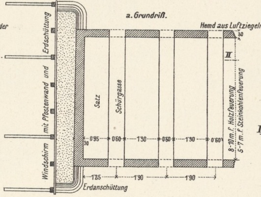
6. Gemauerter Ziegelfofen.
