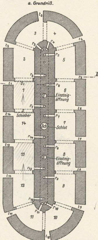
11. Kalkofen mit unterbrochenem Betriebe für Steinkohlenfeuerung.
