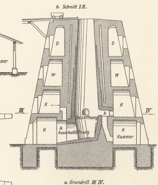
12. Kalkofen mit unterbrochenem Betriebe für Holzfeuerung.
