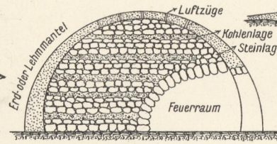
8. Kalkmeiler.
