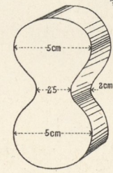
13. Probekörper für Zementproben.
