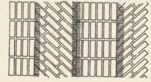
4 1/2. Ziegelschichtung für den Brand.
