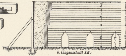
5. Feldofen zum Ziegelbrennen.
