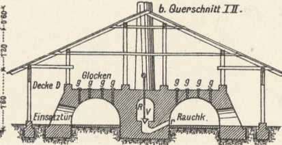
7. Hoffmannscher Ringofen.
