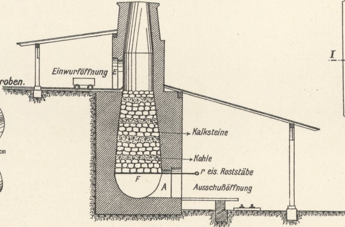
11. Kalkofen mit unterbrochenem Betriebe für Steinkohlenfeuerung.
