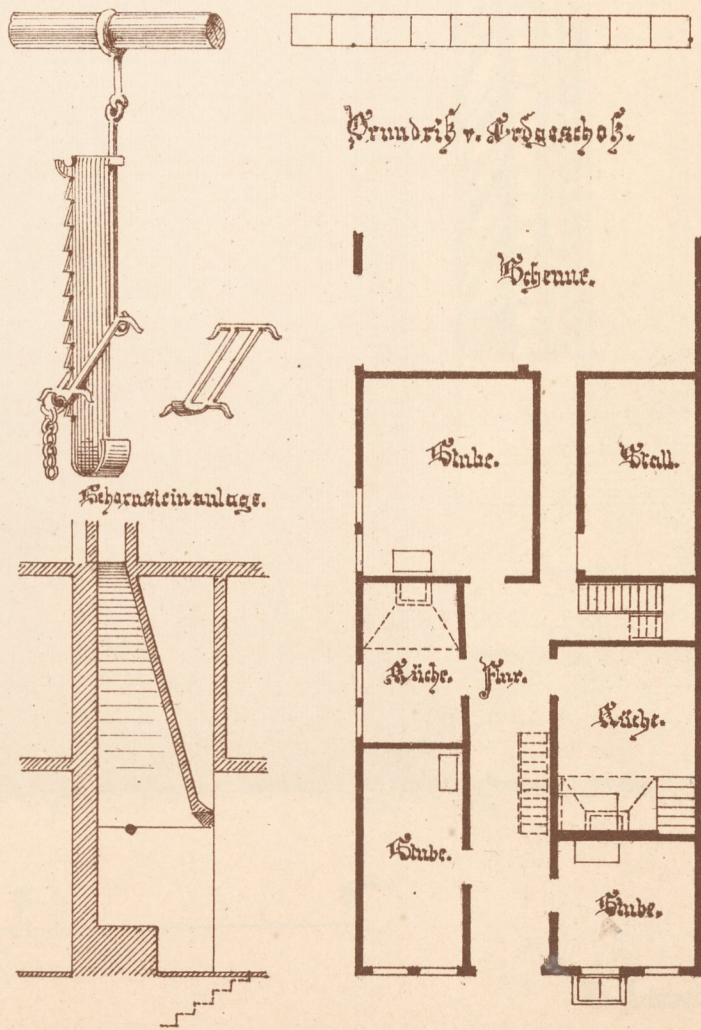
Vorrichtung z. Aufhäng. d. Kocher.
