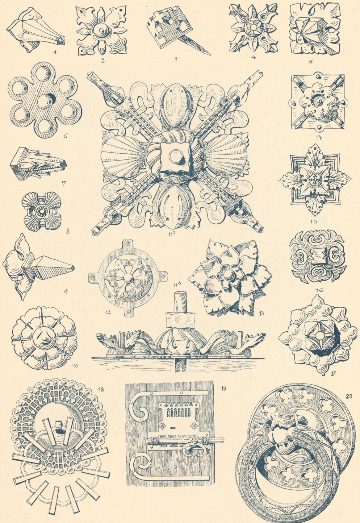
Abb. 138. Geschmiedete Türnägel: 1. Rodez, Kathedrale. — 2. Kastilien. — 3. Salamanca. — 4. Cordova. — 5. Poitiers, Abtei Mortier neuf. — 6. Maurisch. — 7. Tours, Nôtre Dame la riche. — 8. Toledo. — 9. Marseille, S. Victor. — 10. S. Macaire b. Bordeaux. — 11. Spanien, 16. Jahrh. — 12. Rouen, Kathedrale. — 13. Burgos. — 14. Zamora. — 15. Salamanca. — 16. Kastilien, 17. Jahrh. — 17. Kastel S. Germain de Livet bei Lisieux, Küchentür. — 18. Klopfer, Palermo, Palastkapelle (Bronze), 12. Jahrh. — 19. Riegelschloß aus Köln, 15. Jahrh. (Germ. Museum, Nürnberg). — 20. Klopfer, Bayonne, Kathedrale, 13. Jahrh. 19*
