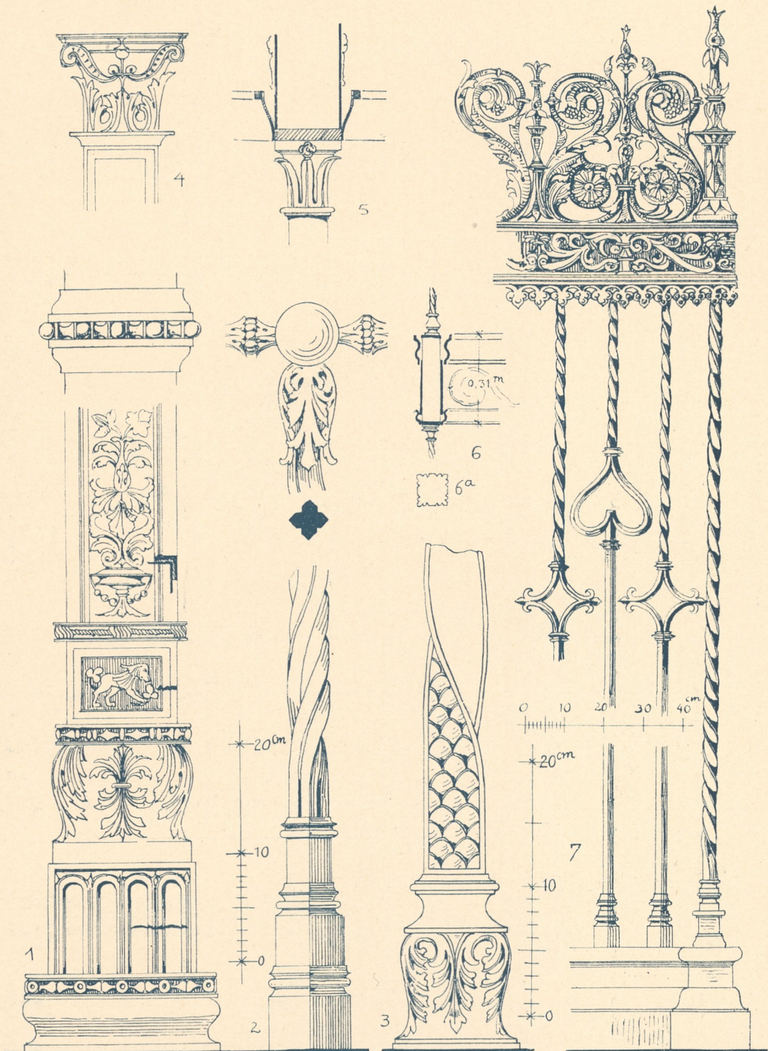
1 u. 2. Kathedrale in Cuenza, Gitter der Capilla major, Einzelheiten vom unteren Teil (vergl. Abb. 130). — 3, 4, 5. Kathedrale in Cuenza, von dem Gitter hinter dem Hochaltar, von Sancho Muñoz. — 6. Kathedrale in Toledo, Gitter der Heil. Geist-Kapelle, von Domingo Cespedes (1529), Friesprofil; 6a. Profil der gedrehten Stäbe. — 7. Kathedrale in Sigüenza, Kapellengitter (1530).
