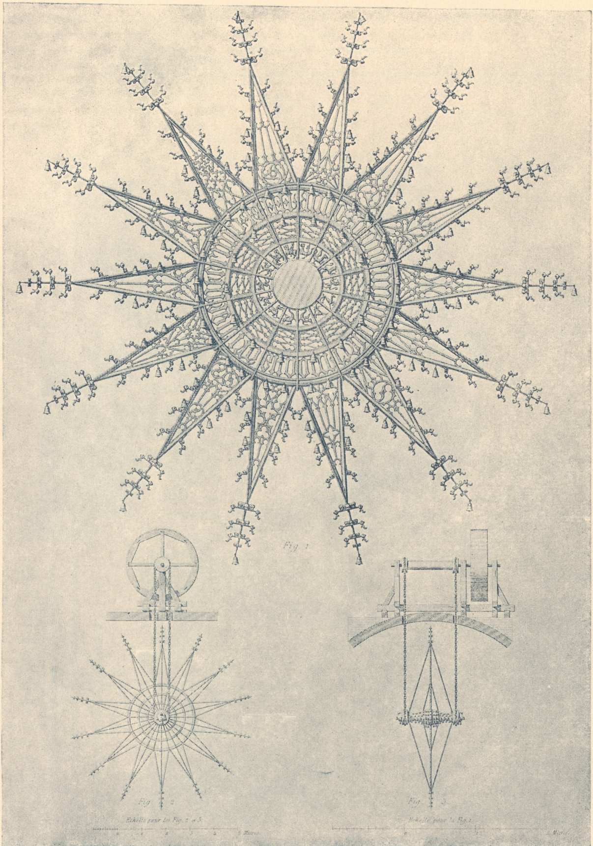
Abb. 83. Glockenrad (Schmiedeeisen und Bronze) im Dom zu Fulda (1415). (Aus Gaillhabaud, l'Architecture du Ve au XVIIe siècle.)
