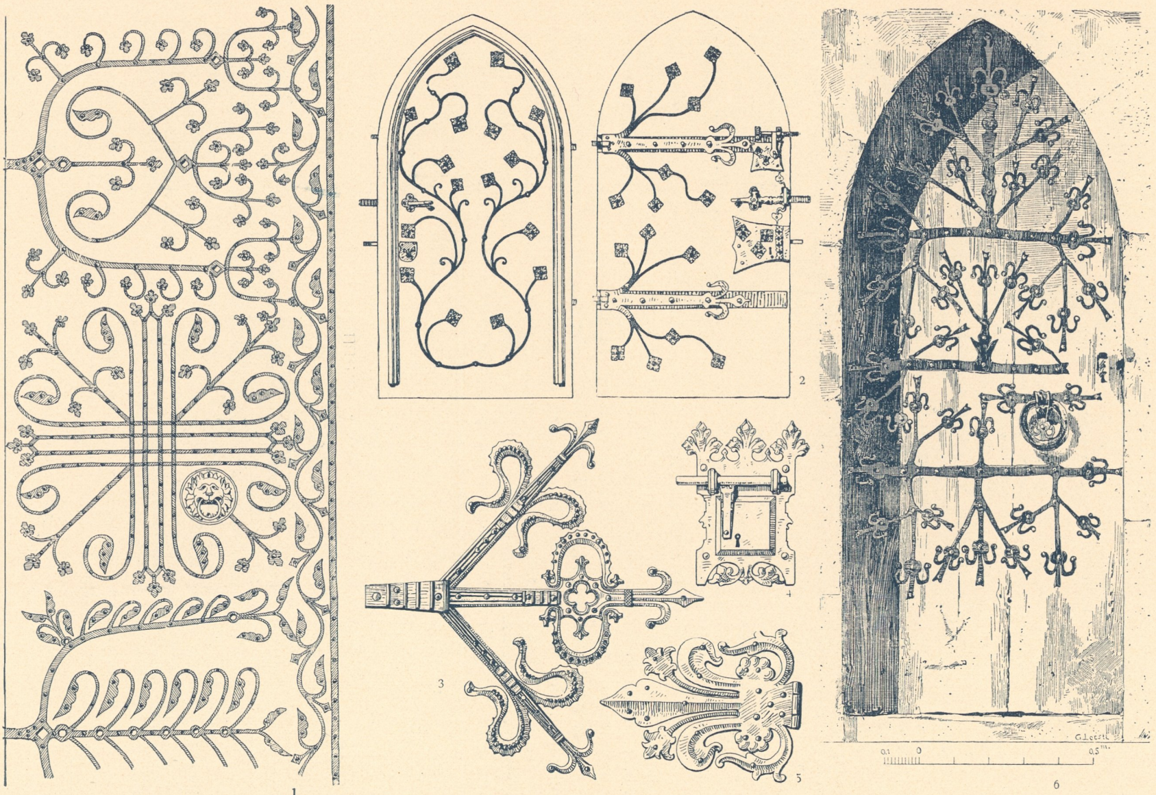
Abb. 55. 1. Beschlag der Westtür der Elisabethkirche in Marburg, 1283. — 2. Türe im Germ. Museum, Nürnberg, 1,90 m hoch, 15. Jahrh. — 3. Türband, Kirche zu Viersen b. Köln, Anf. 15. Jahrh. — 4. Riegelschloß aus Bingen a. Rh. — 5. Türband, Kathedrale zu Antwerpen, um 1400. — 6. Sakristeitür der Stadtkirche zu Weilderstadt (aus „Kunst- und Altertumsdenkmale im Königreich Württemberg“).
