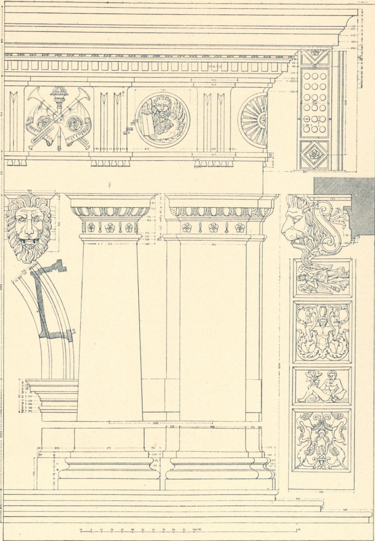
Fig. 376. Bibliothek San Marco in Venedig. Details des Erdgeschosses (n. Raschdorff, Venedig, Tafel 60).
