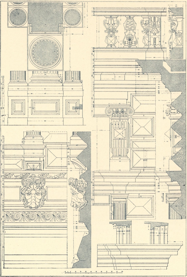
Fig. 372. Palazzo Pesaro in Venedig. Details vom Erd- und Zwischengeschoss (n. Raschdorff, Venedig, Taf. 92).
