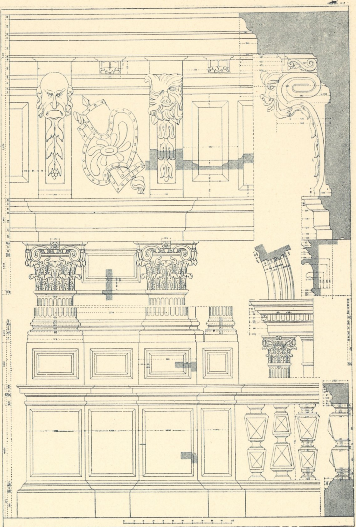
Fig. 373. Palazzo Pesaro in Venedig. Details vom 2. Obergeschoss (n. Raschdorff, Venedig, Taf. 93.)
