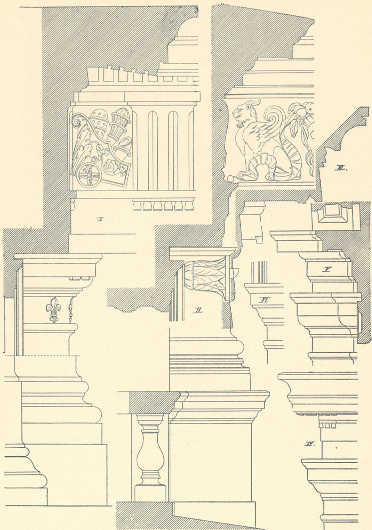
Fig. 367. Palazzo Farnese in Rom. Säulenstellungen, Hauptgesimse und Kämpfergesimse (n. Letarouilly).
