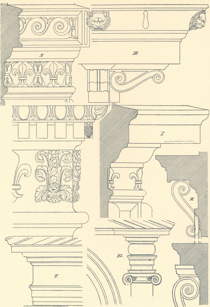
Fig. 366. Palazzo Farnese in Rom. Gurt- u. Hauptgesimse, Fensterkrönungen (n. Letarouilly).
