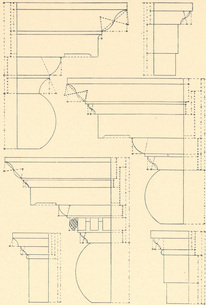
Fig. 362. Fenster und TürGESIMSE (n. Palladio).
