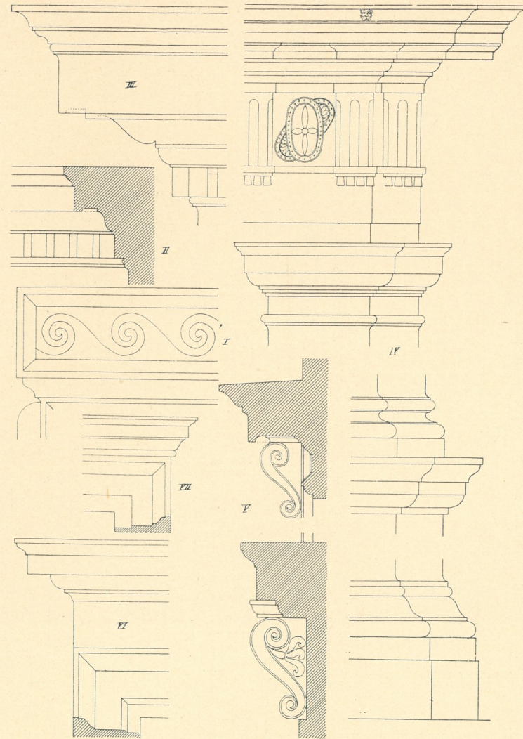
Fig. 363. Palazzo Palma in Rom Gurtgesimse, Hauptgesimse und Fenster pp. (n. Letarouilly).
