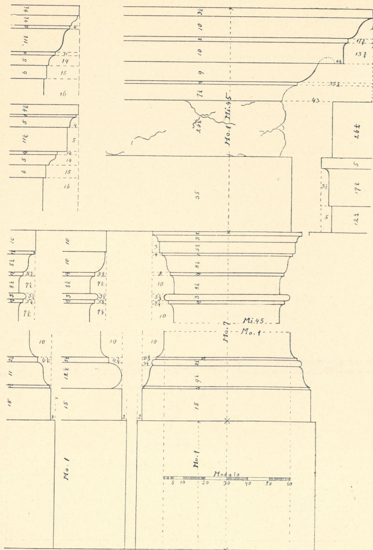
Fig. 354. Toskanische Säulenordnung und zwei Kämpfer-Profile (n. Palladio).
