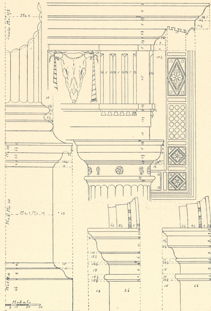
Fig. 355. Dorische Säulenordnung und zwei Kämpferkapitäl mit Volute (n. Palladio).
