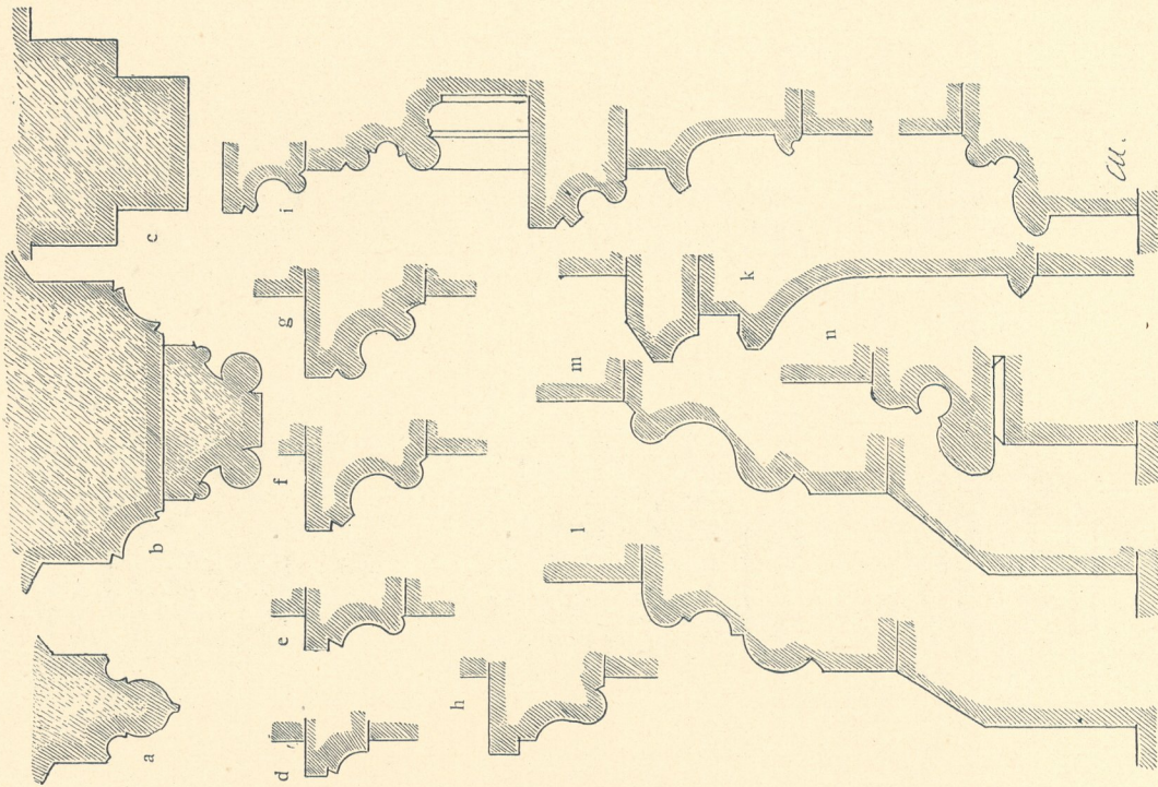
Fig. 306. Marienkirche zu Gelnhausen. a, b, c) Gewölbegurten, d—h) Gurtgesimse, i) Zwerggalerie am Chor, m, k) von Balkons, e) Sockel am Chor, m) Sockel am Schiff.
