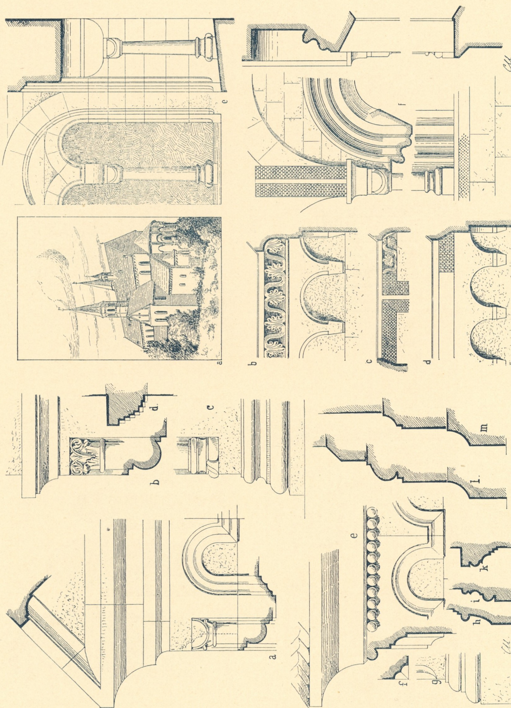
Fig. 220. a) Klosterkirche zu Hamersleben, b) Hauptgesimse des Mittelschiffs, c) Hauptgesimse des Chores, d) Hauptgesimse der kleinen Absis, e) Turmfenster, f) Chorfenster.
