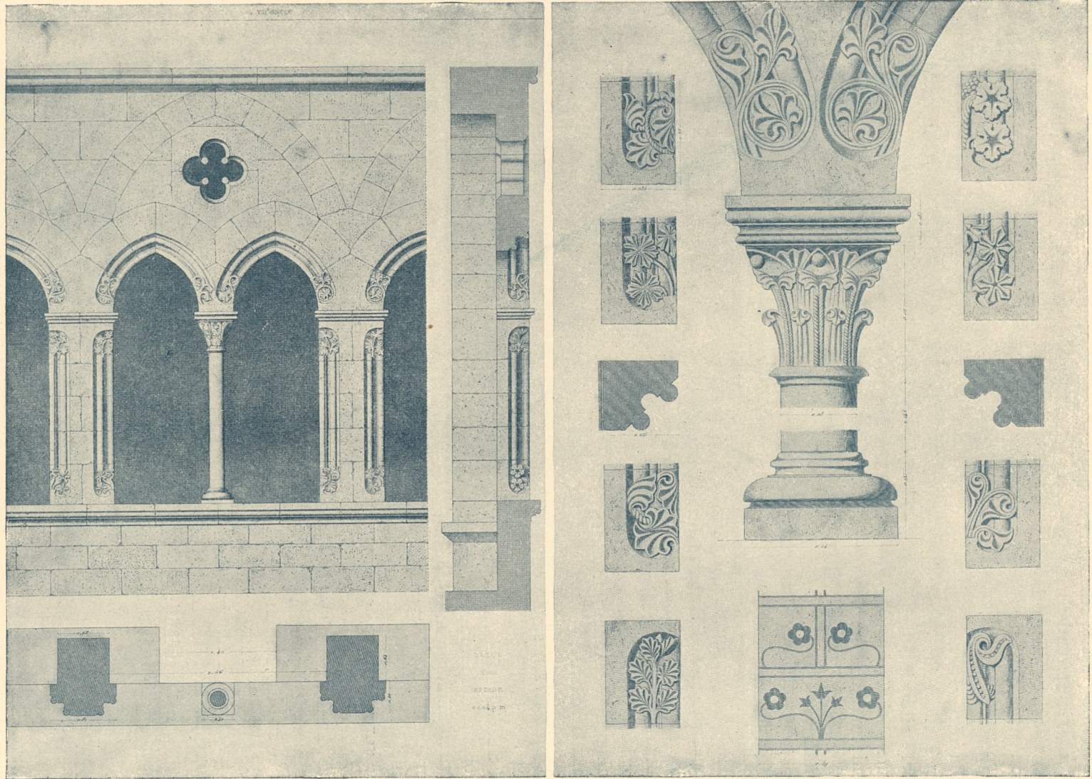
Fig. 205. Details von einem Hause in Figeac, Frankreich (n. Verdier et Cattois, Bd. I Seite 150, 151).
