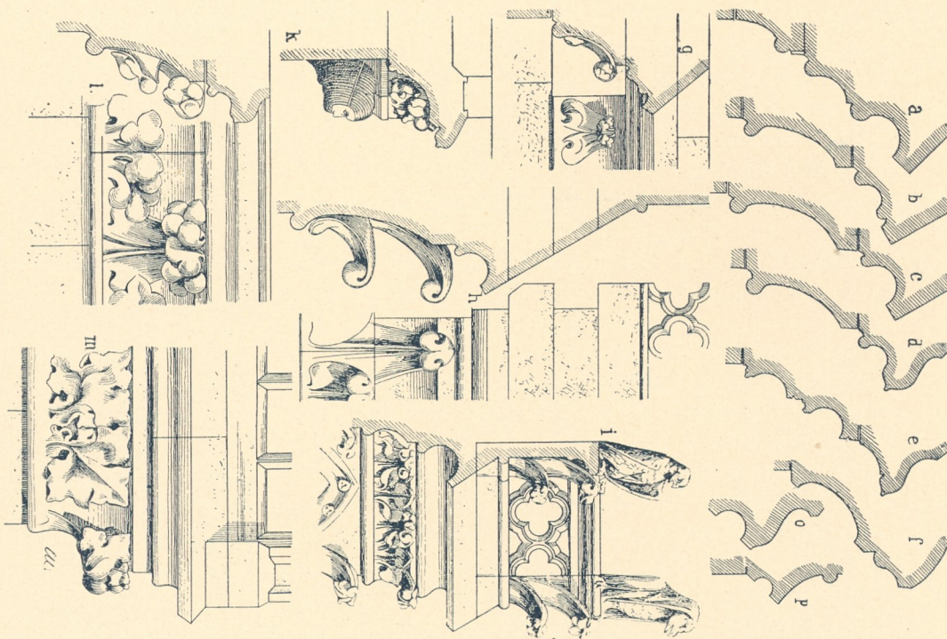
Fig. 180. Gotische Hauptgesimse a, b, c) XIII. Jahrh., d) XIV. Jahrh., e) XV. Jahrh. f, o, p) XVI. Jahrh. (n. Viollet-le-Duc).
