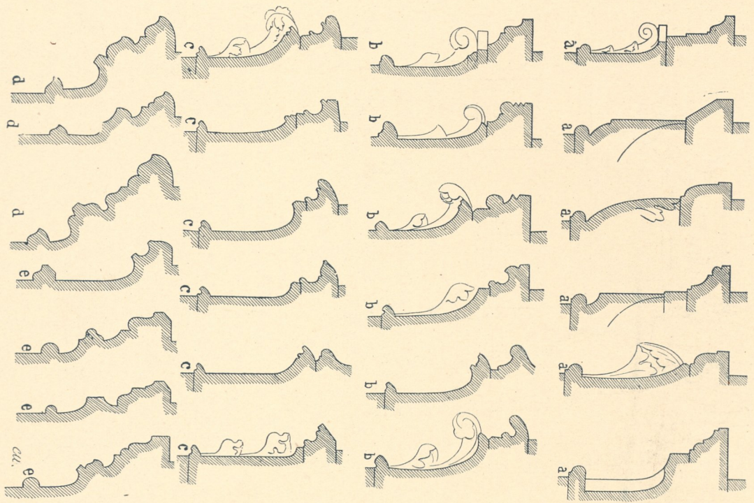
Fig. 178. Säulenkapitälé. a) XI.-XII. Jahrh., b) XIII. Jahrh., c) XIV.-XV. Jahrh., d) Englisch „Decorated style“, e) Englisch „Perpendicular style“.
