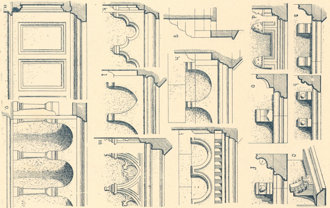
Fig. 179. Romanische Hauptgesimse aus dem XI.-XII. Jahrhundert.
