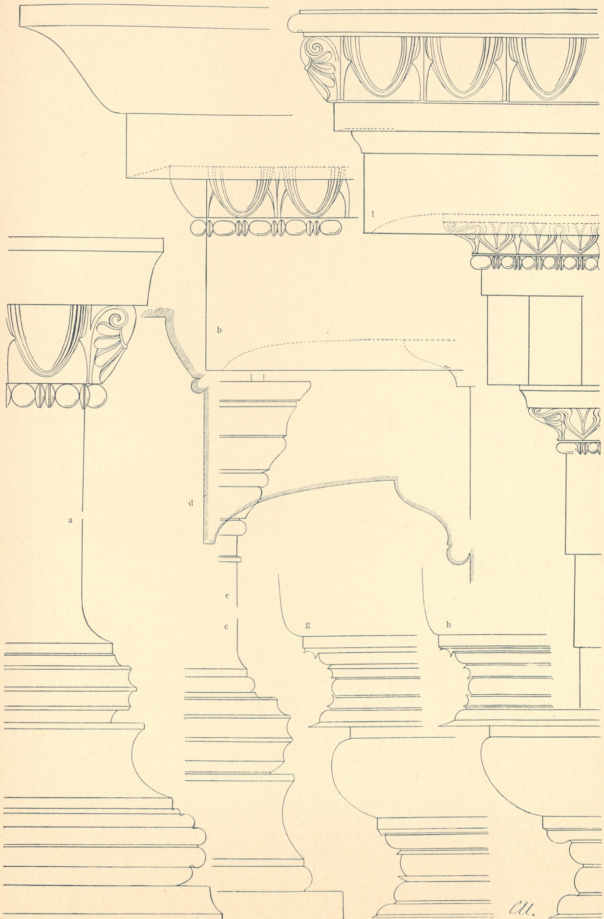
Fig. 48. a) b) c) Nike-Tempel. a) Sockelgesimse. b) Hauptgesimse. c) Säulenfuß. d)–h) Erechtheion.
