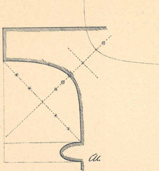
Fig. 11. Konstruktion der Hohlkehle vom Tempel Medinet Haboo nach Pennethorne.
