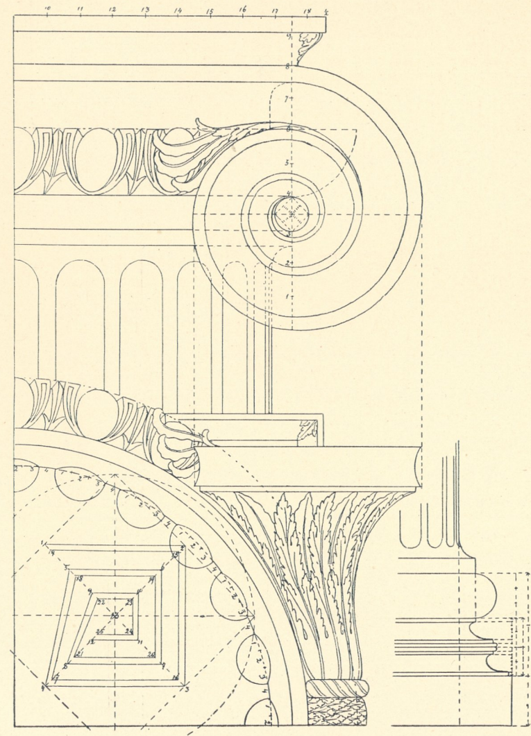
Fig. 357. Jonisches Kapitäl mit Untersicht und Schema der Schnecke und jonischer Posis (n. Palladio).
