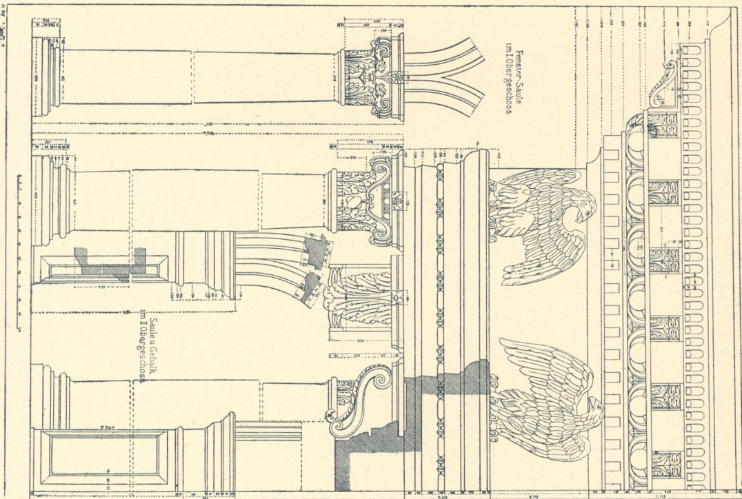
Fig. 371. Palazzo Vendramin Calergi in Venedig. Details vom 2. Obergeschoss (n. Raschdorff, Venedig, Tafel 35).
