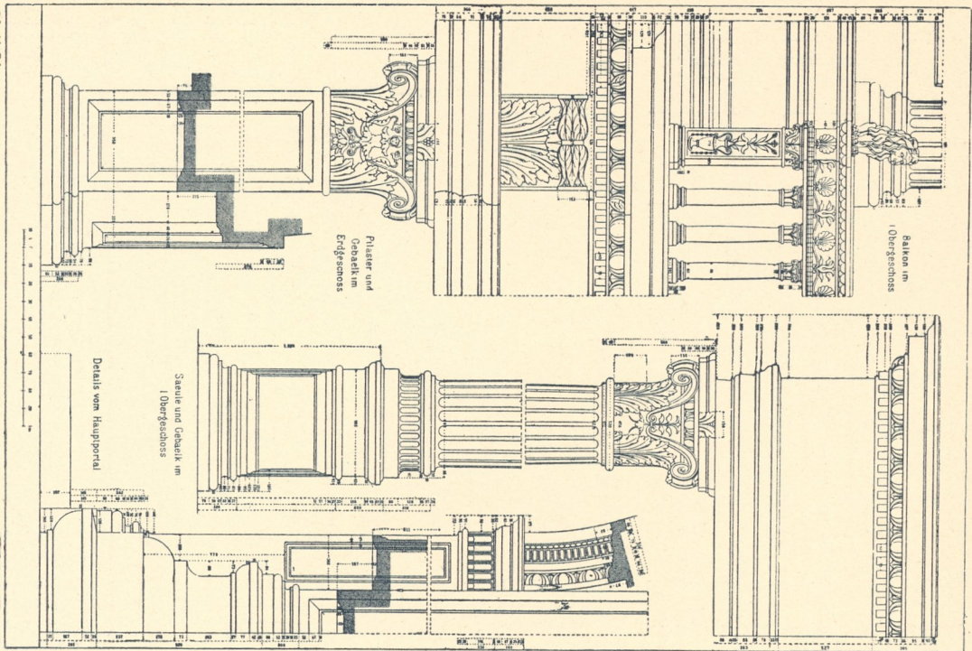
Fig. 370. Palazzo Vendramin Calergi in Veneug. Details vom Erd- und I. Obergeschoss (n. Raschdorff, Venedig, Tafel 34).
