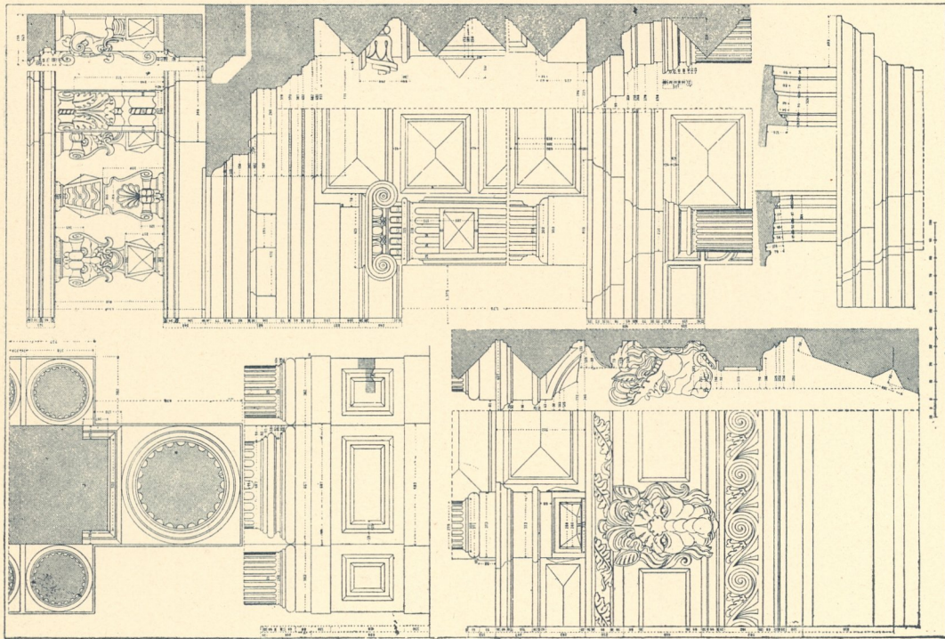
Fig. 372. Palazzo Pesaro in Venedig. Details vom Erd- und Zwischengeschoss (n. Raschdorff, Venedig, Taf. 92.)
