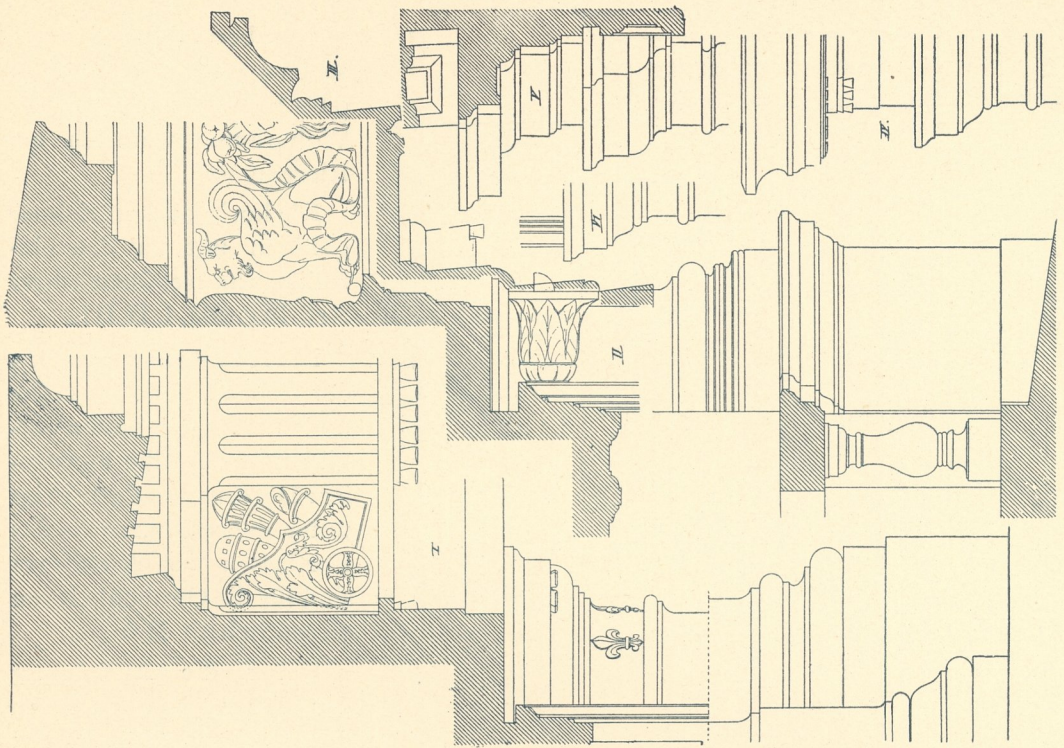
Fig. 367. Palazzo Farnese in Rom. Säulenstellungen, Hauptgesimse und Kämpfgesimse (n. Letarouilly).
