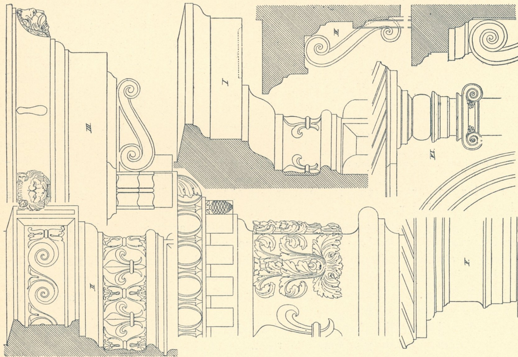
Fig. 366. Palazzo Farnese in Rom. Curt- u. Hauptgesimse, Fensterkrönungen (n. Letarouilly).
