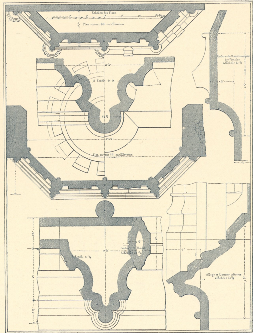
Fig. 293. Détails zu dem Erker neben der Kathedrale zu Wells
