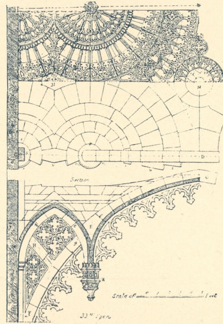
Fig. 297. Die Gewölbe über der Kapelle Heinrichs des VII. in West- minster-London. (The Architect 1900.)
