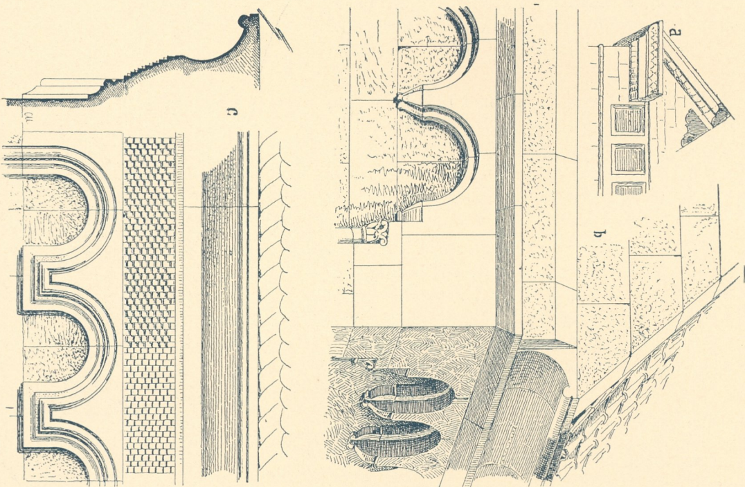
Fig. 214. a) Giebelösung der Kirche zu Sinzig, b—c) Hauptgesimse des Mittelschiffs und der Seitenabsiden an der Stiftskirche zu Königsalter.
