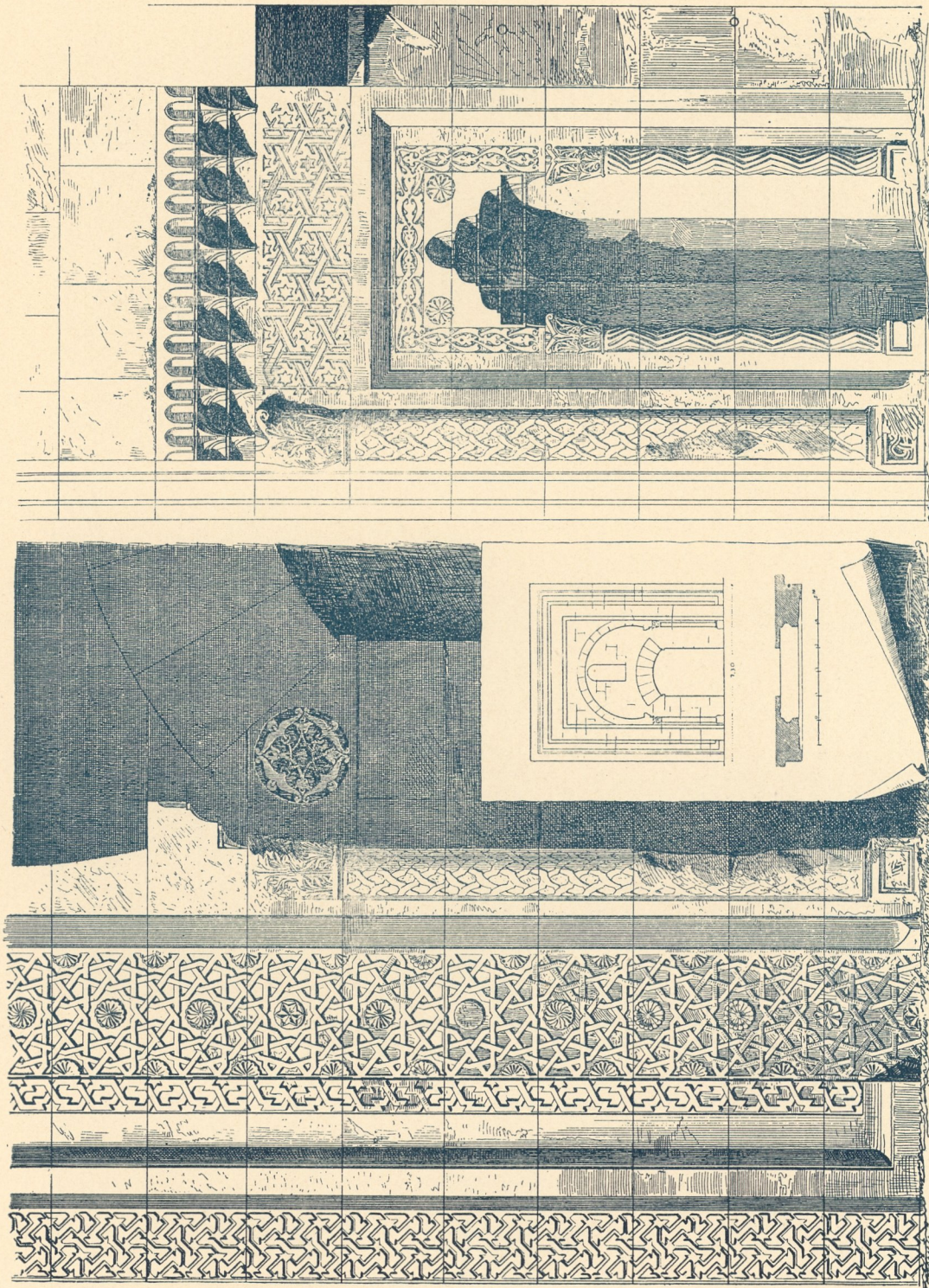
Fig. 167. Portal und Querschnitt eines Madrasse (n. Lanckoronski, Pamphylien Bd. I pag. 28 und 29 im Text).
