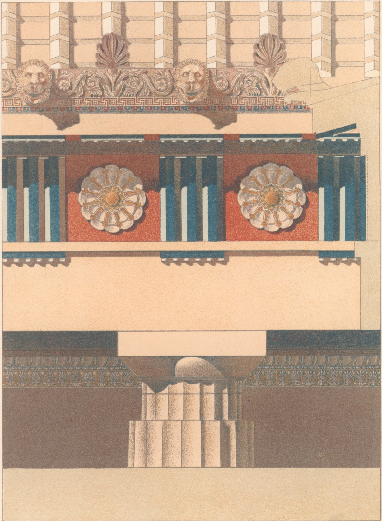
Fig. 45 und 58. Aeussere Säulenstellung des Tholos des Asklepios zu Epidauros. (n. Defrasse und Lechat. Pl. VI.)
