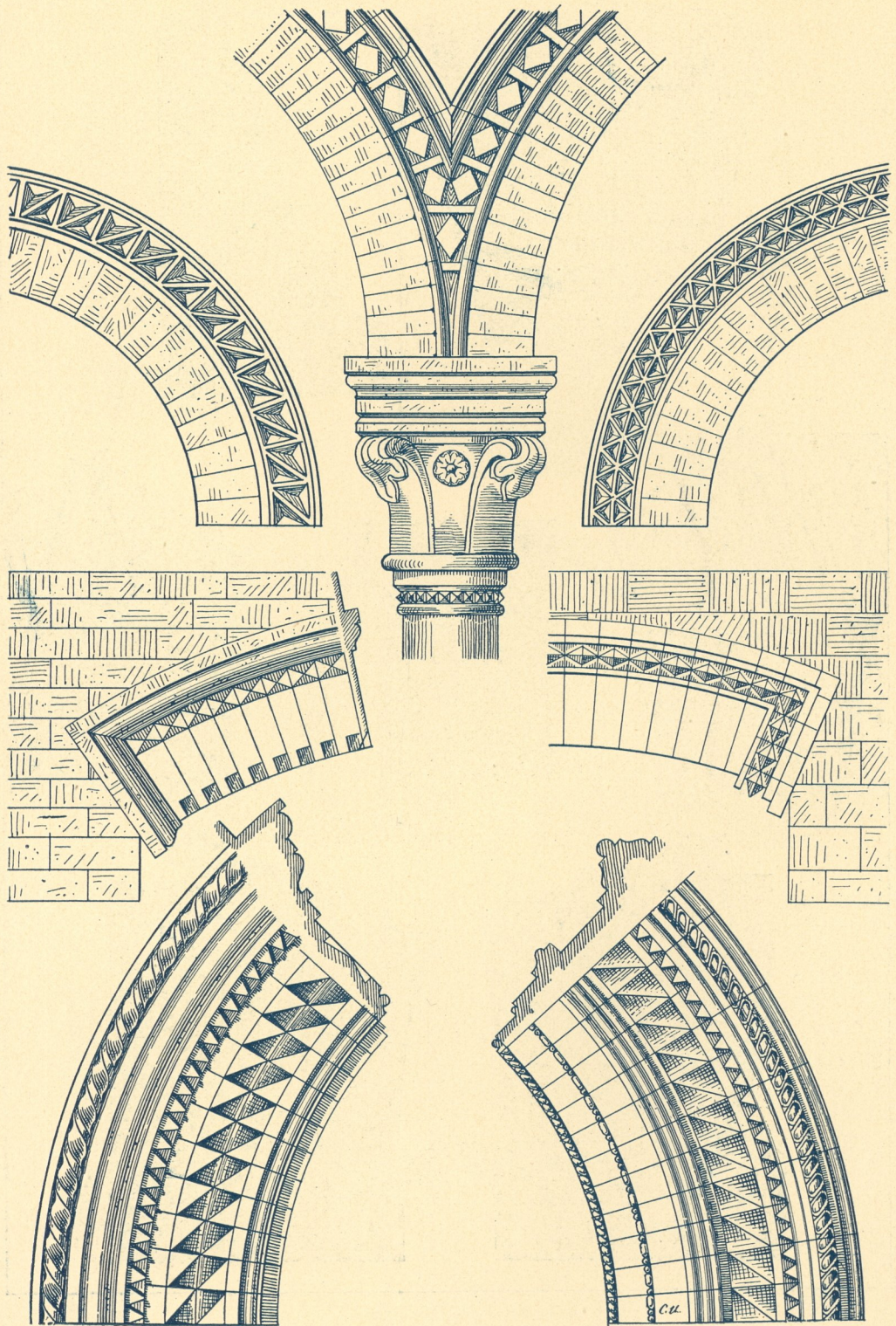
Fig. 34. Archivolten aus Ferrara, Bologna und Faenza.
