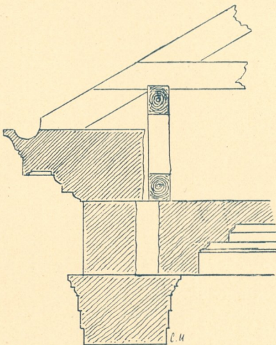
Fig. 306. Hauptgesimse mit Fries und Deckenlage im Innern.
